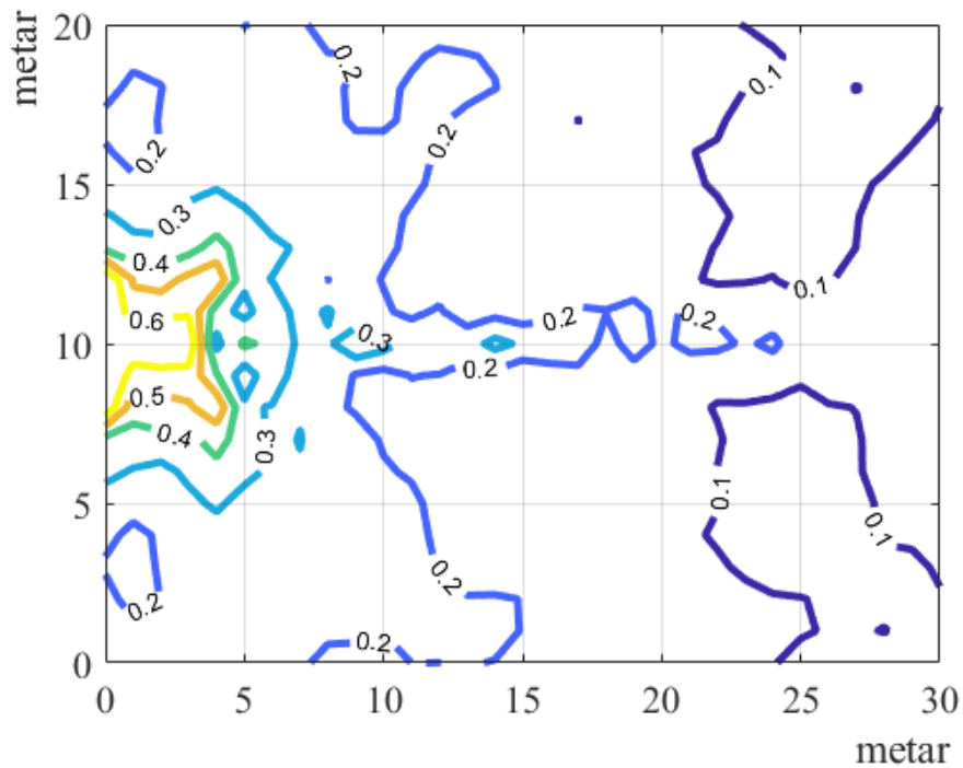
Prilog 18 Polje koeficijenta transmisije za val valne visine 0,9 m i perioda 4,16 s; djelomično uronjena grupa propusta (W2) postavljena na koordinati (0,10) i os propusta je paralelna s apcisonom (Slika 63)
