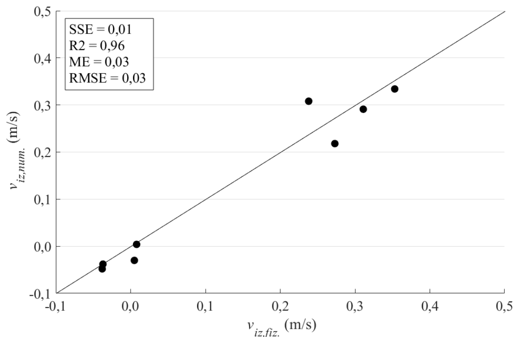
Slika 61 Validacija brzina vode dobivenih kroz numerički model ( v_{iz,num} ) u odnosu na mjerene vrijednosti u okviru laboratorijskih ispitivanja ( v_{iz,fiz} ) bilježene pomoću ADV uređaja (Slika 15)
