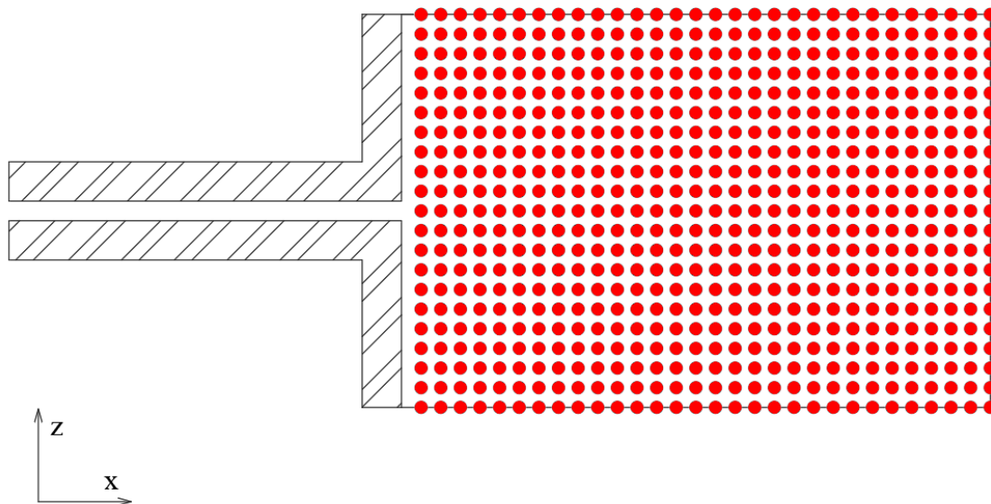
Slika 37 Pozicije numeričkih sonde unutar zaštićenog akvatorija dužine 3 m i širine 2 m (ne uključuje dio numeričke mreže gdje se obavlja relaksacija vala odnosno umirenje valne energije); mreža postavljena numeričkih sonde se sastoji od 30 stupaca i 21 reda
