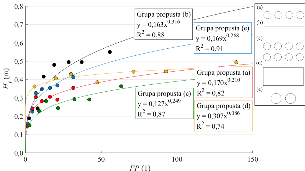
Slika 78 Odnos fluks parametra ( FP ) i srednje transmitirane valne visine unutar prethodno definiranog područja ( H_t ) (Slika 63) za pojedine testove po pojedinim ispitivanim oblikovanjima grupe propusta provedene u okviru numeričkog modeliranja; u prirodnom mjerilu
