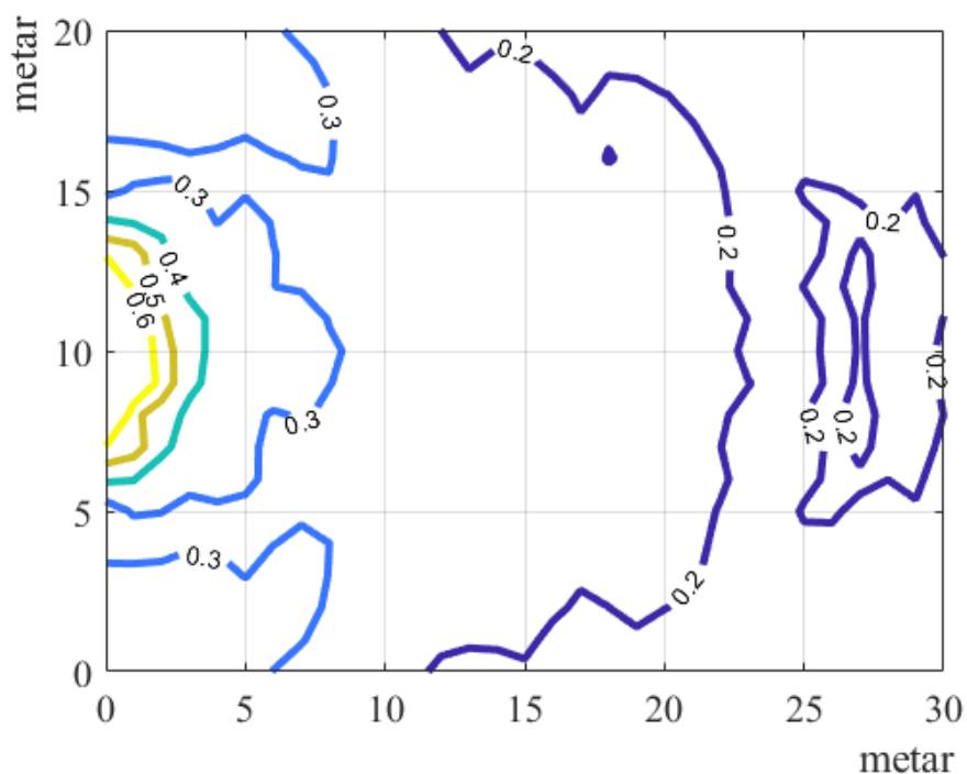
Prilog 40 Polje koeficijenta transmisije za val valne visine 0,9 m i perioda 4,16 s; djelomično uronjena grupa propusta (W2) postavljena na koordinati (0,10) i os propusta je paralelna s apcisonom (Slika 63)
