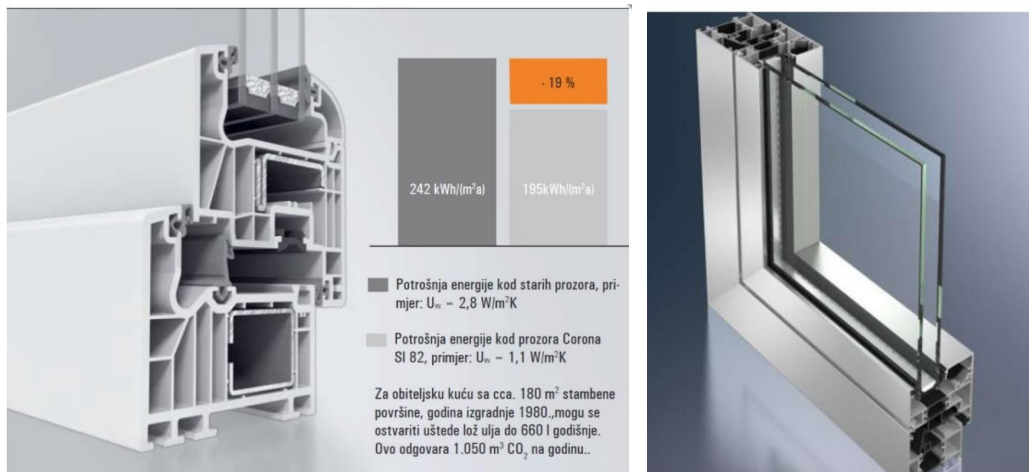
Slika 23: PVC i aluminijски Schuco prozori
