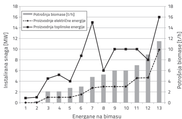
Slika 13. Potrošnja biomase po satu ovisno o instaliranoj snazi [5]
