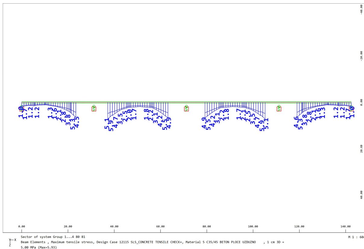
Slika 6.12. Prikaz najvećih vlačnih naprezanja u betonskoj ploči
