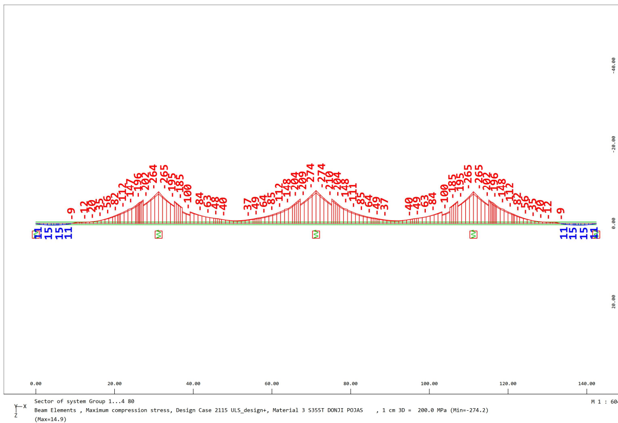
Slika 6.16. Najveće tlačno naprezanje u donjem pojasu
