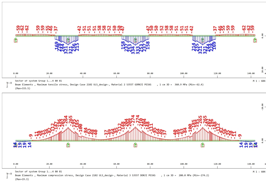
Slika 6.14. Najveće vlačno napreznje gornjeg pojasa i najveće tlačno napreznje donjeg pojasa
