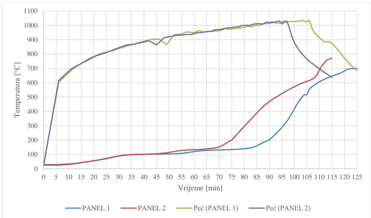
Slika 58. Spoj 3. sloja ploča i PUR pjene na izloženoj strani – termočlanak T14
