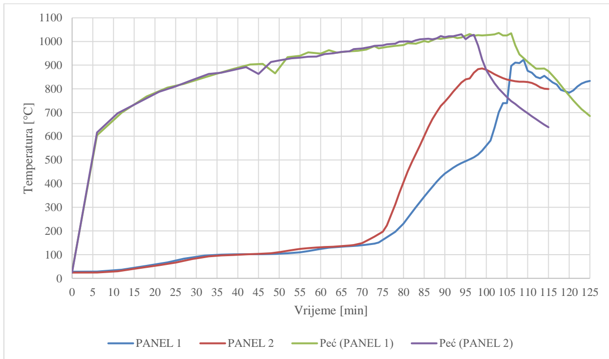
Slika 61. Spoj 3. sloja ploča i PUR pjene na izloženoj strani – termočlanak T18
