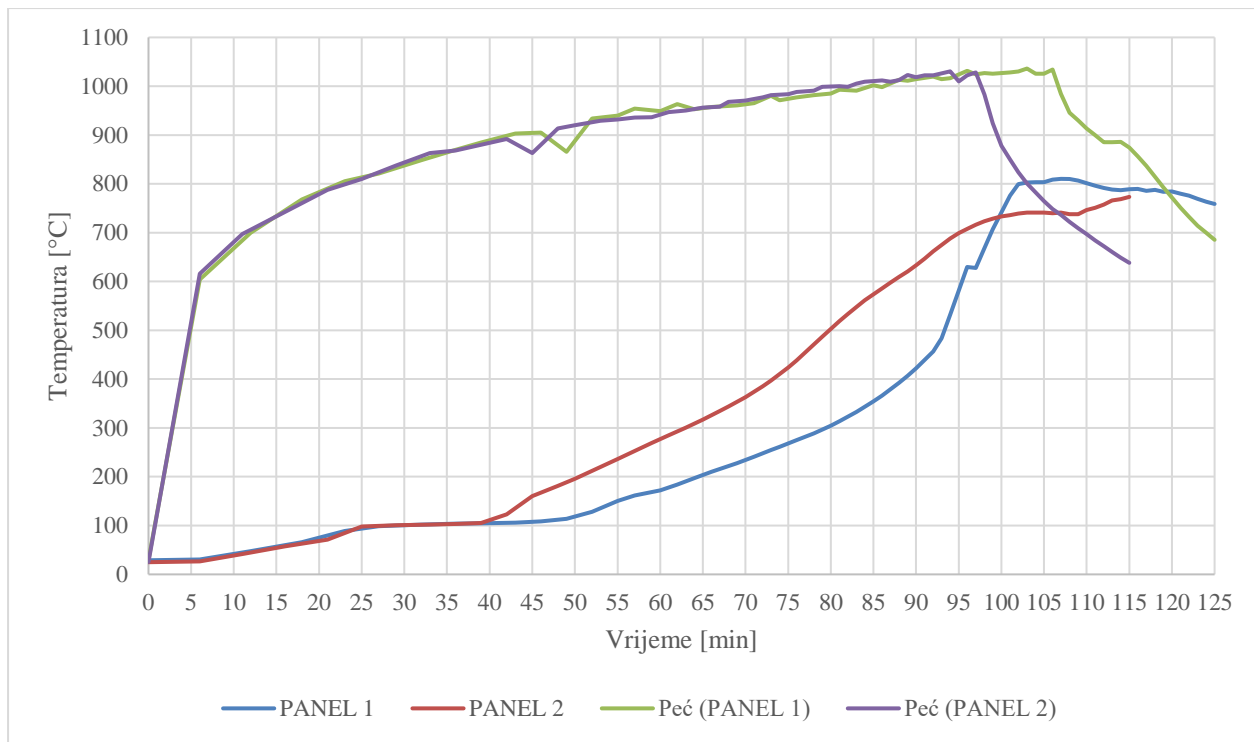
Slika 54. Spoj 2. i 3. sloja ploča na izloženoj strani – termočlanak T8
