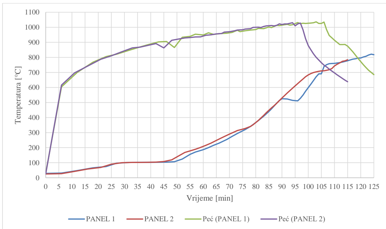
Slika 55. Spoj 2. i 3. sloja ploča na izloženoj strani – termočlanak T9
