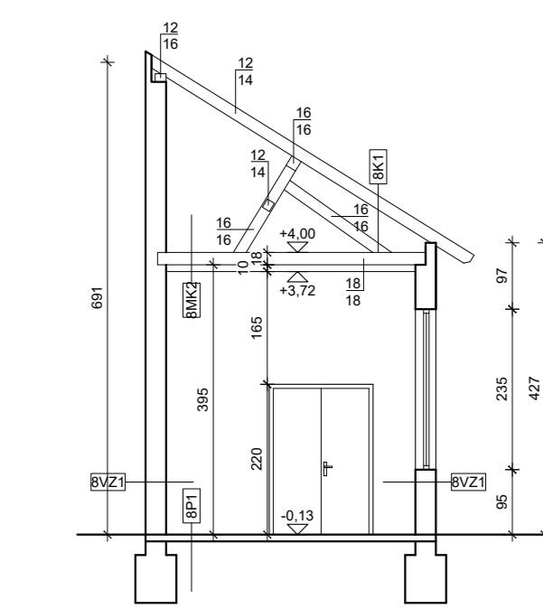
ZGRADA 8 PRESJEK 4-4
