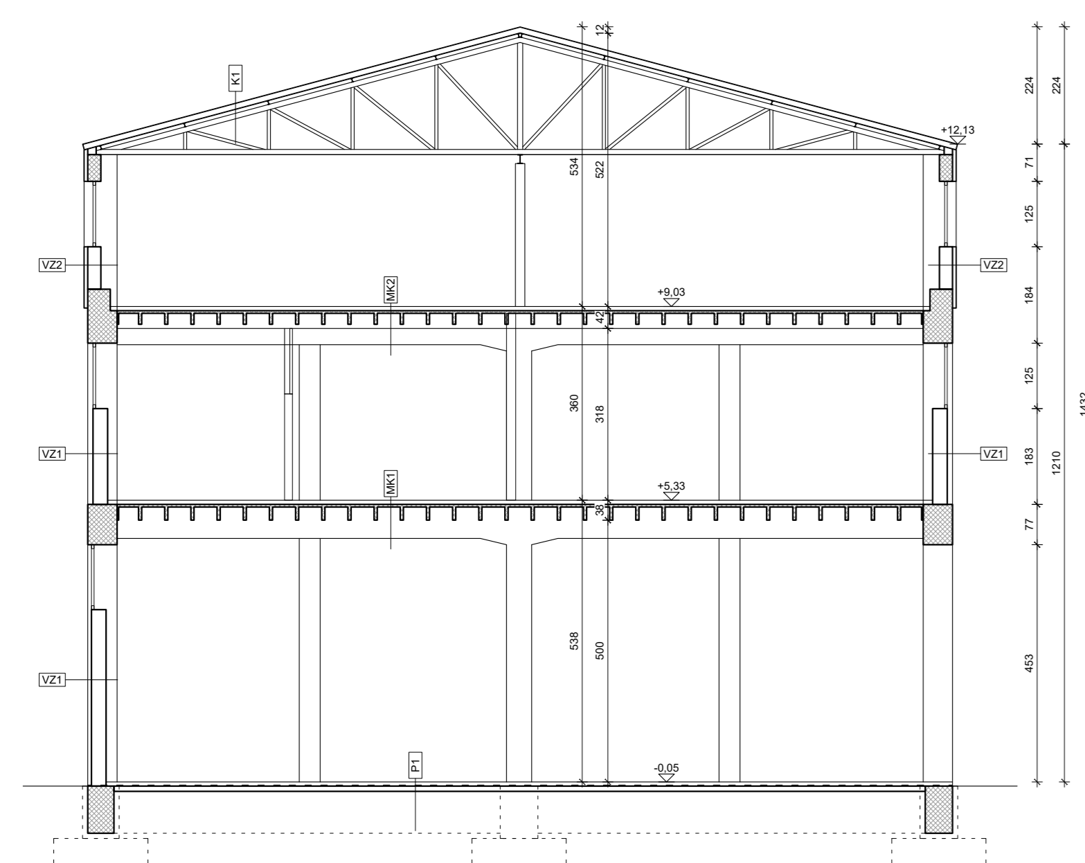
PRESJEK C-C
