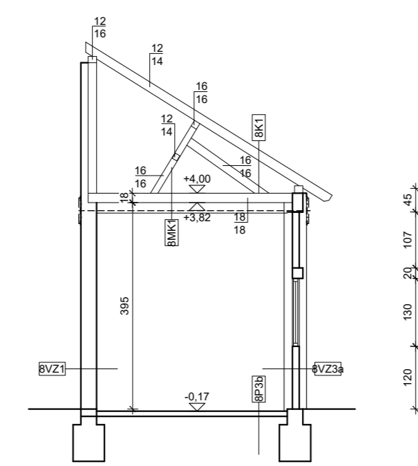
ZGRADA 8 PRESJEK 6-6
