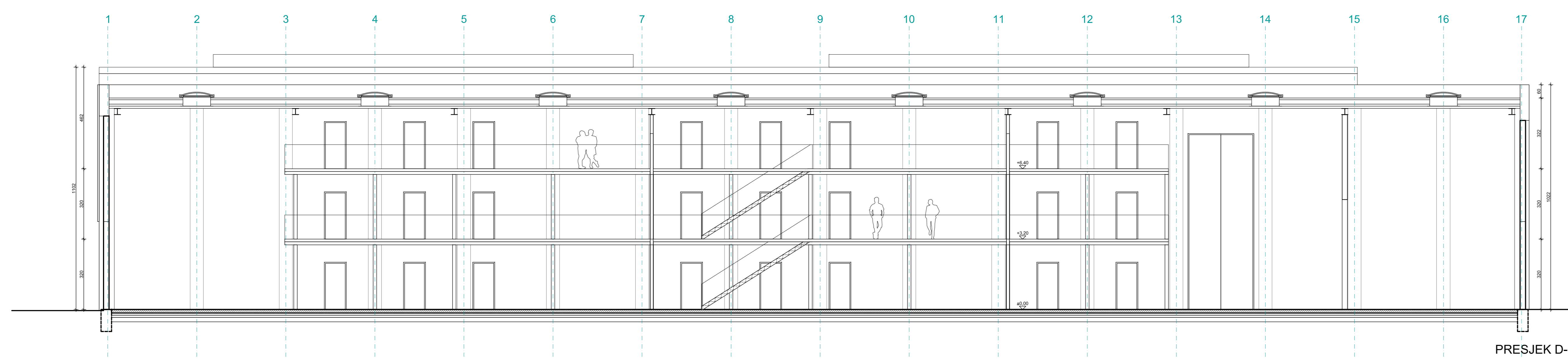
PRESJEK D-D
