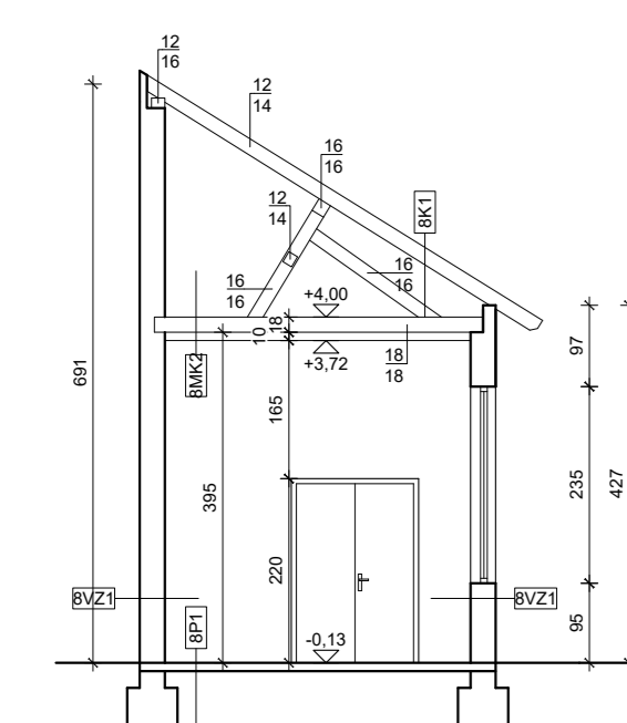
ZGRADA 8 PRESJEK 4-4
