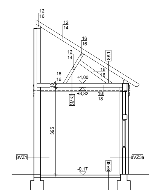
ZGRADA 8 PRESJEK 6-6
