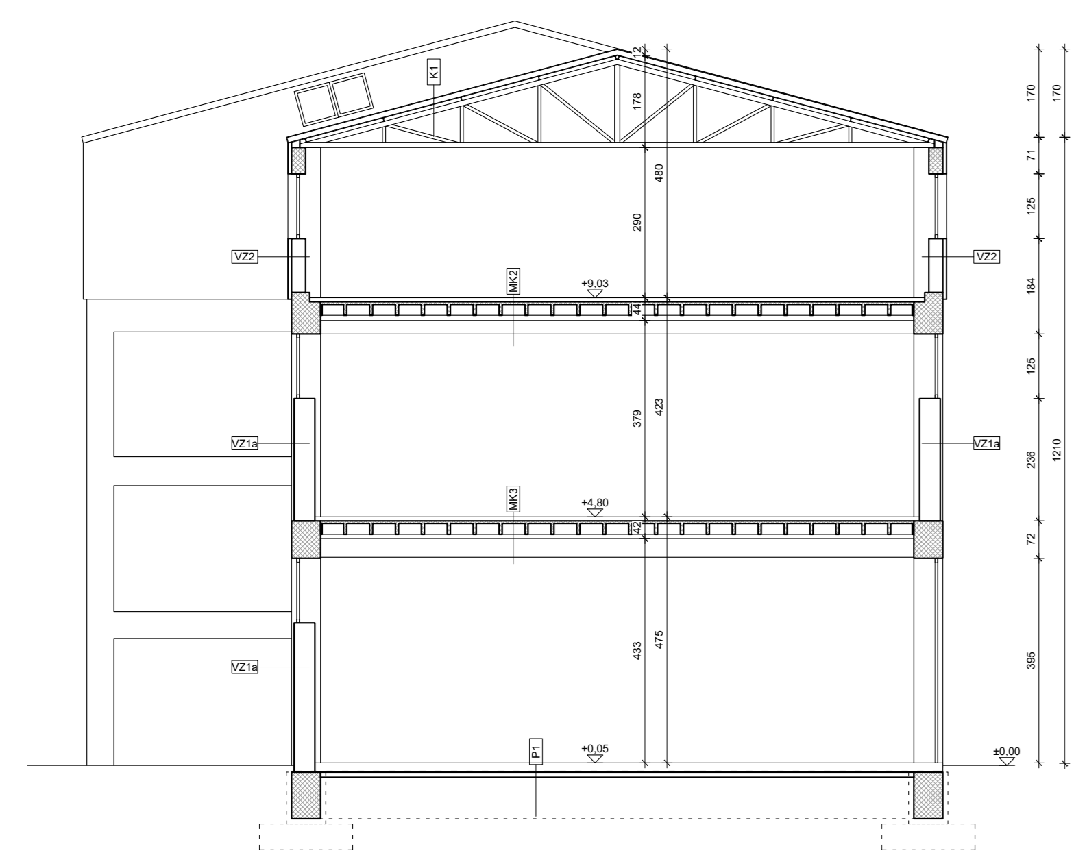
PRESJEK C-C
