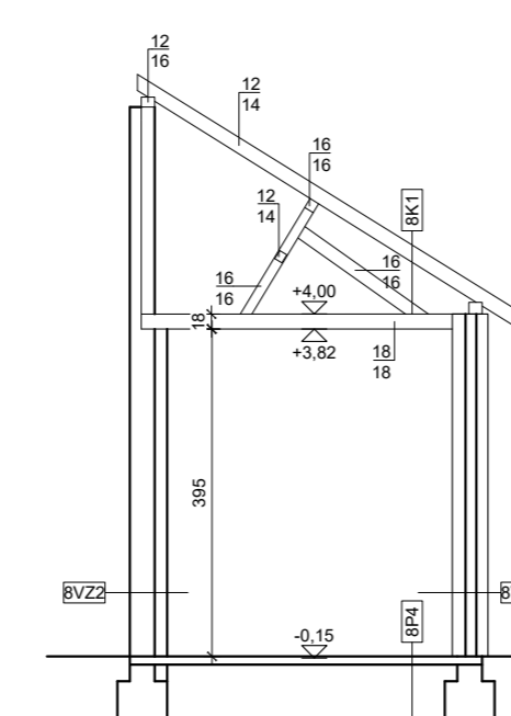
ZGRADA 8 PRESJEK 7-7
