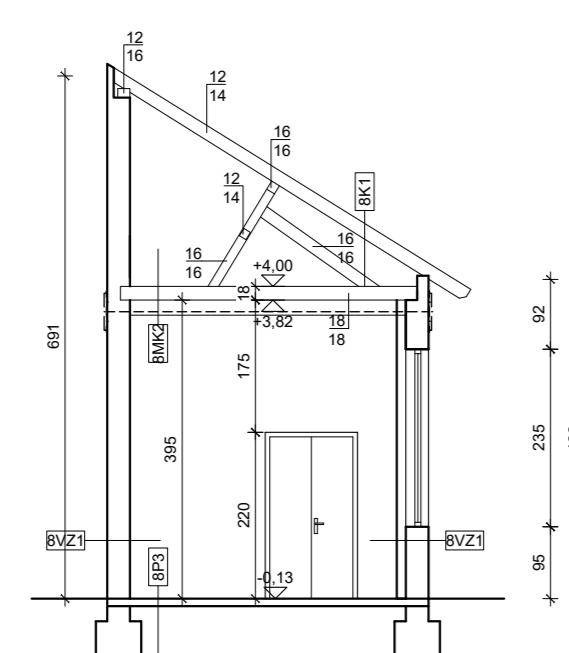
ZGRADA 8 PRESJEK 5-5
