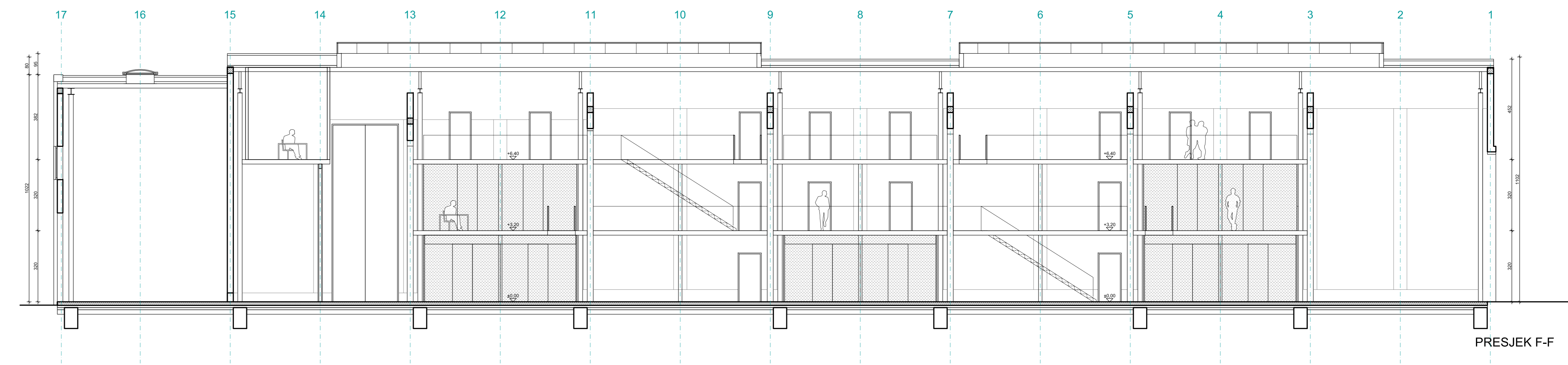
PRESJEK F-F
