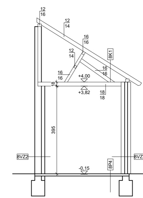
ZGRADA 8 PRESJEK 7-7
