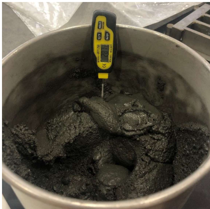
Slika 10. Prikaz mjerenja temperature betona u svježem stanju mješavine M-1
