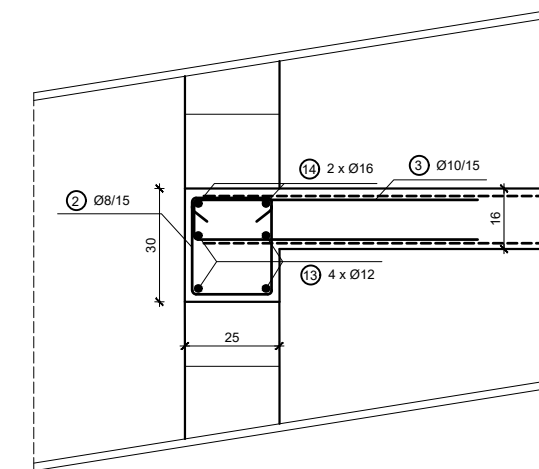
Presjek P6 MJ 1:20
