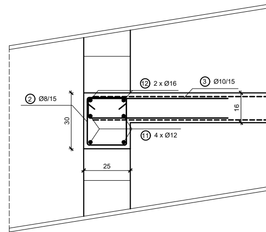
Presjek P9 MJ 1:20
