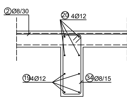
PRESJEK 17-17 M=1:25
