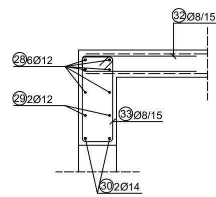
PRESJEK 24-24 M=1:25
