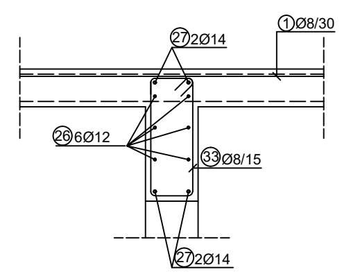
PRESJEK 20-20 M=1:25
