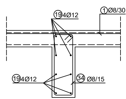
PRESJEK 21-21 M=1:25
