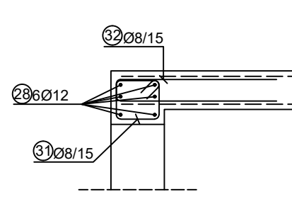
PRESJEK 23-23 M=1:25
