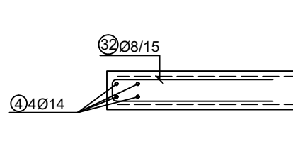
PRESJEK 22-22 M=1:25
