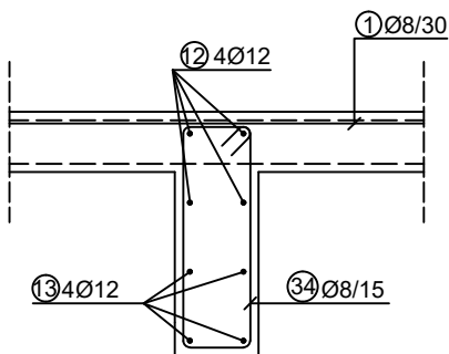
PRESJEK 5-5 M=1:25
