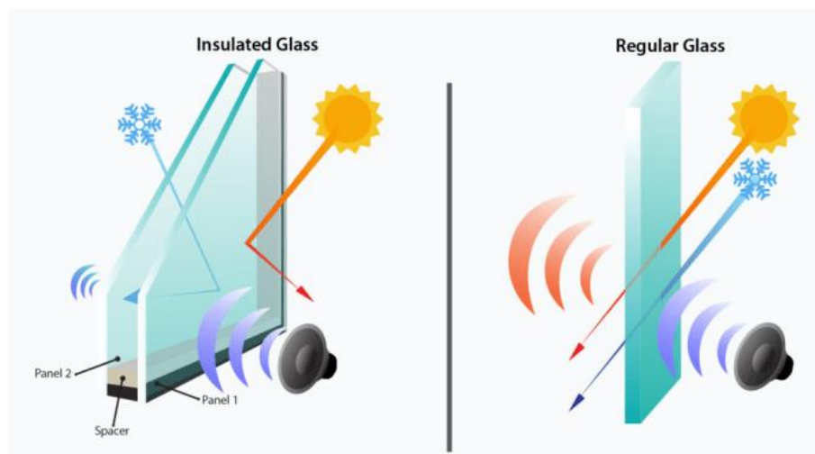
Slika 18. Izolirano ostakljenje
