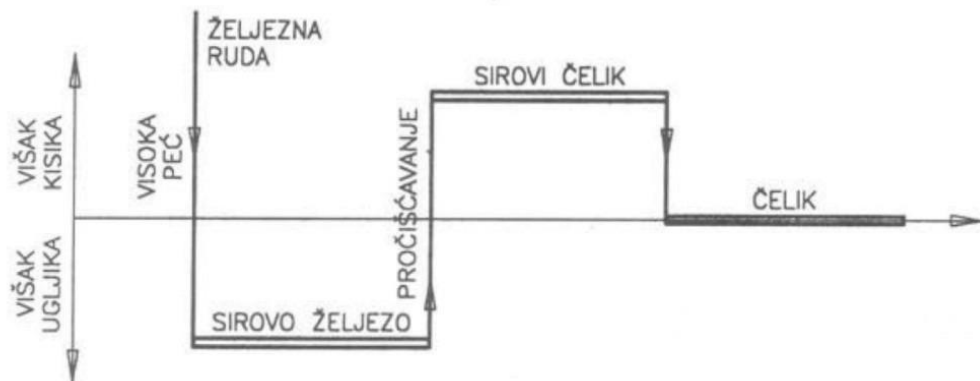
Slika 1. Shematski prikaz proizvodnje čelika
