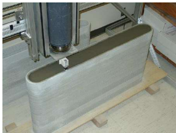
Slika 3. Proces punjenja okvira
