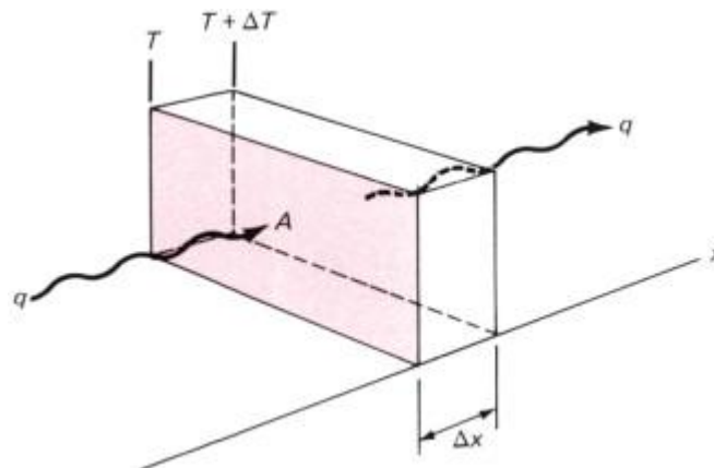
Slika 22: Fourierov zakon [80]
