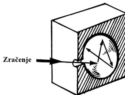
Slika 5: Crno tijelo [51]
