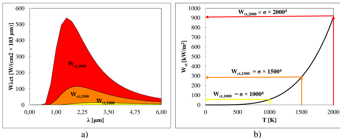
Slika 10: Stefan-Boltzmannov zakon
