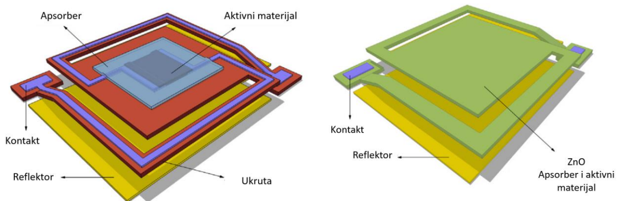
Slika 4: Mikrobolometar –Shematski prikaz klasičnog (a) mikrobolometra, (b) jednoslojnog mikrobolometra [48]
