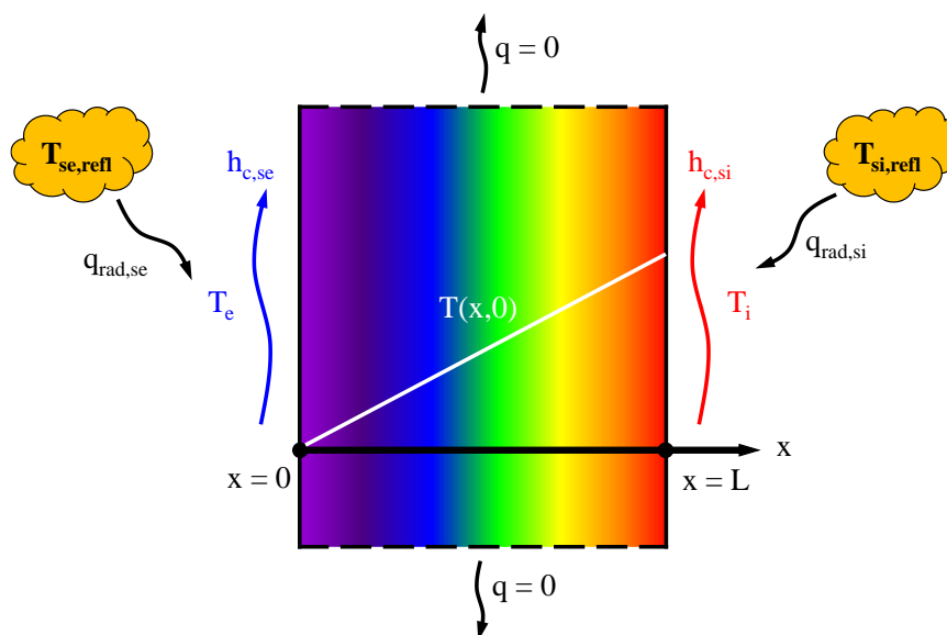
Slika 23: 1D provođenje topline
