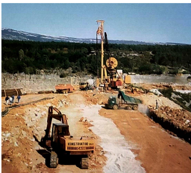
Slika 8 - Radovi na sanaciji desnog boka brane [7].
