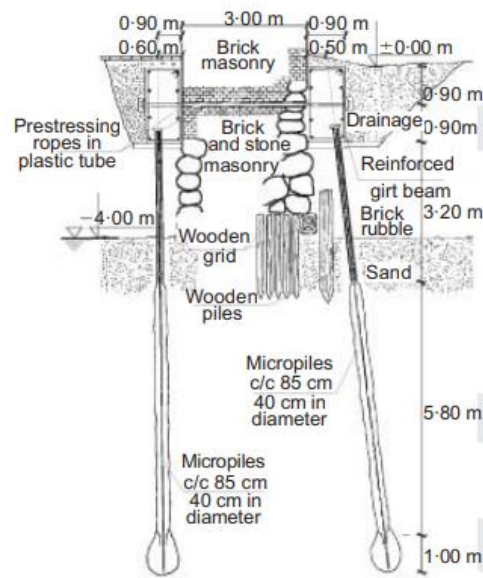
Slika 17 Potpora pomoću pilota dvorca Malbork
