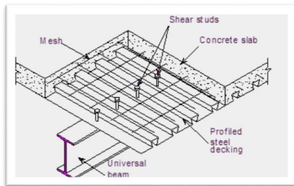
Slika 19 Kompozitna ploča s profiliranim metalnim podom [20]
