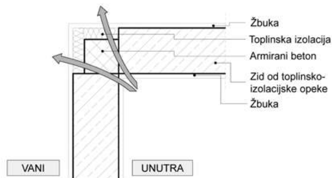
Slika 13. Toplinski most
