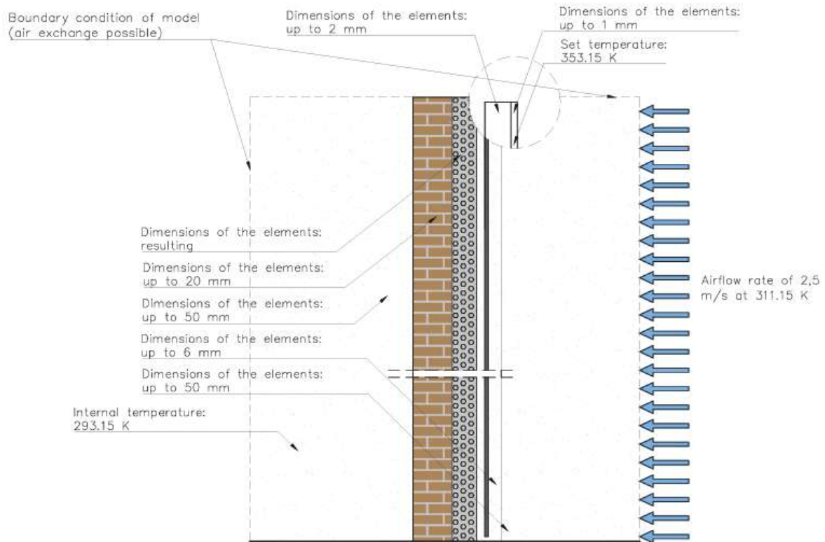
Slika 29. Numerički model zatvorene ventilirane fasade
