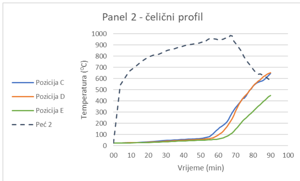
Slika 35 Prikaz razvoja temperature kroz čelični profil
