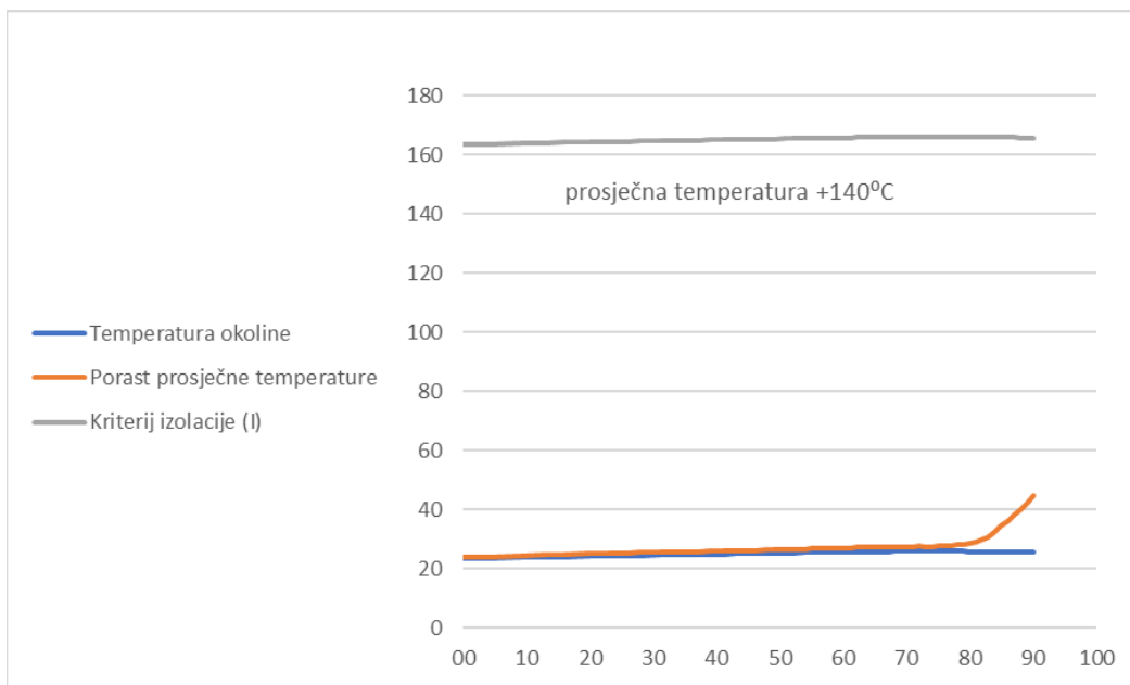
Slika 31 Prikaz razvoja temperature na neizloženoj strani Panela 2
