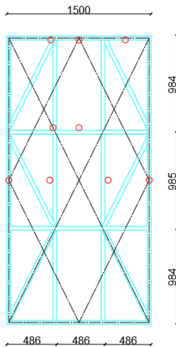
Slika 12 prikaz položaja termočlanaka za mjerenje srednje temperature na neizloženoj strani (+ \Delta 180K )
