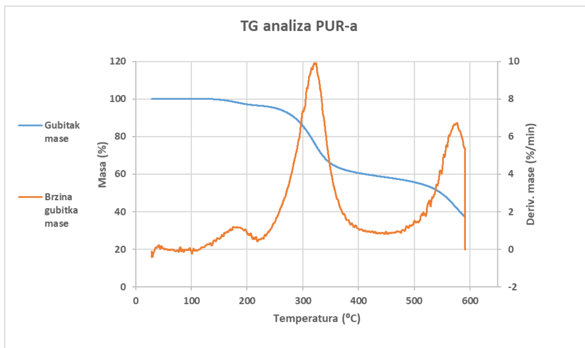
Slika 16 Termogram PUR-a
