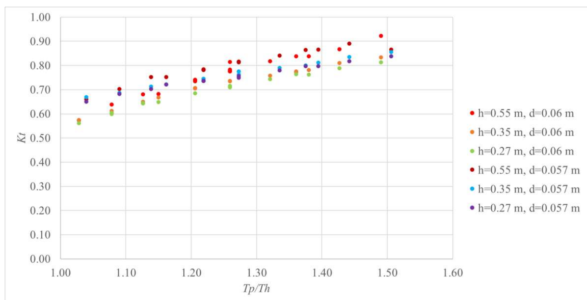
Slika 21 Mjereni koeficijenti transmisije Kt u odnosu na omjer vršnog perioda vala i prirodne oscilacije uzdizanja plutajućeg lukobrana
