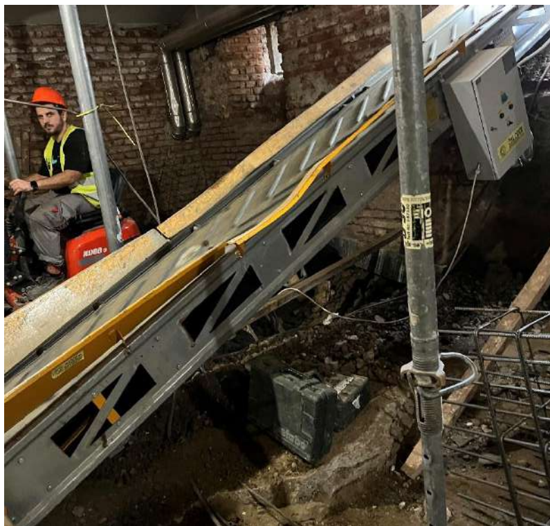
Slika 26 Transportna traka
