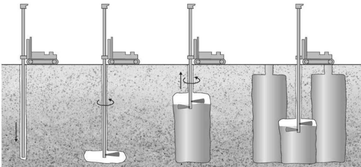
Slika 12 Redoslijed izvođenja mlaznog injektiranja (Arapov i dr., 2009.)
