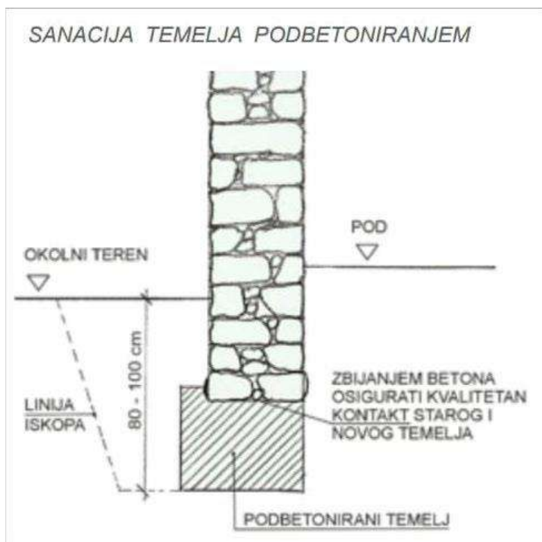
Slika 7 Podbetoniravanje temelja (Puljiz, 2020.)
