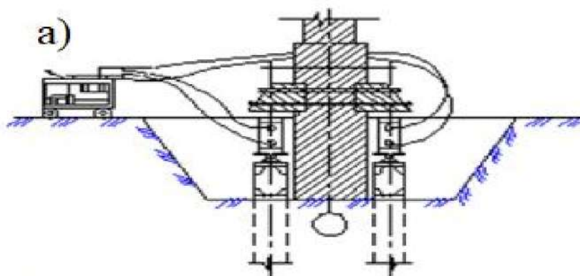
Slika 11 Ojačanje temelja pomoću višeslojnih pilota (Cherney, 2020.)
