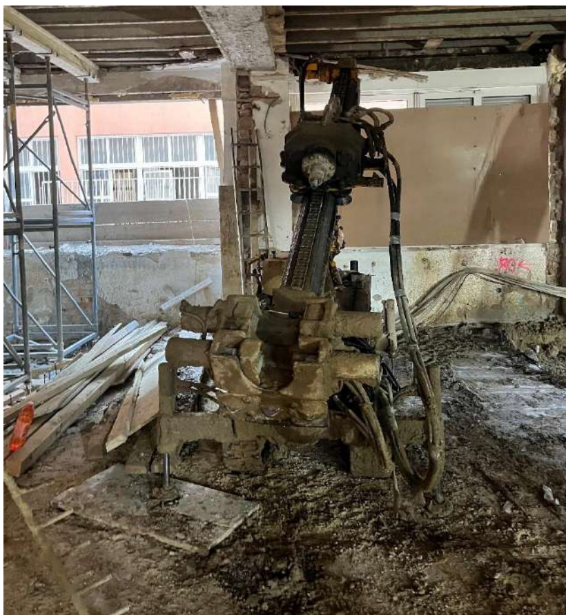
Slika 33 Stroj za bušenje
