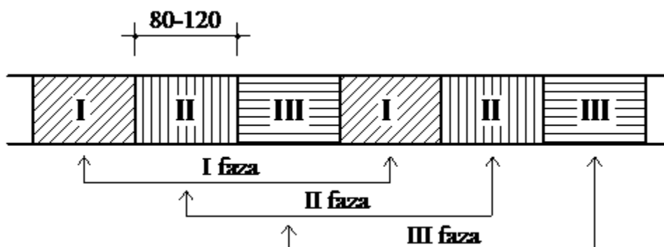
Slika 8 Podbetoniranje po fazama (Stevanović i dr., 2014.)
