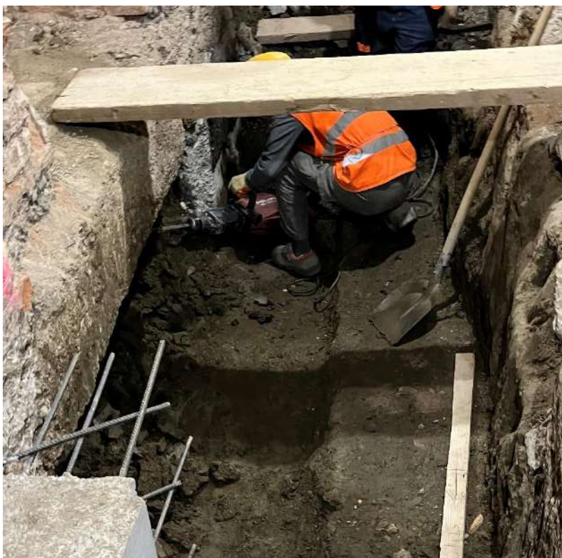
Slika 25 Ručni iskop
