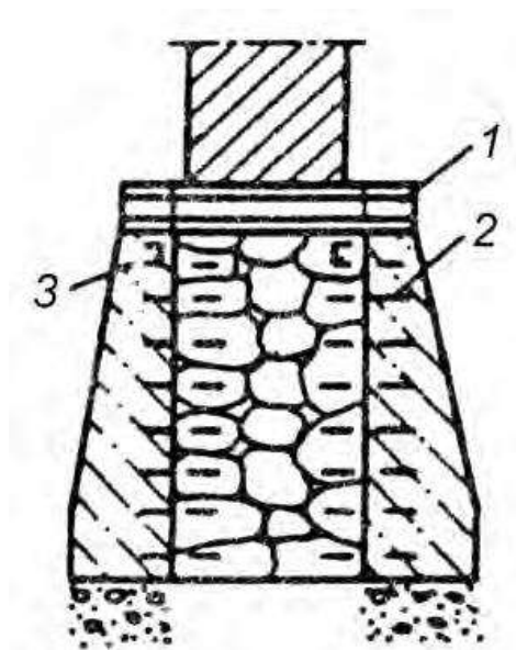
Slika 6 Kombinirano ojačanje i proširivanje temelja (Stevanović i dr., 2014.)
