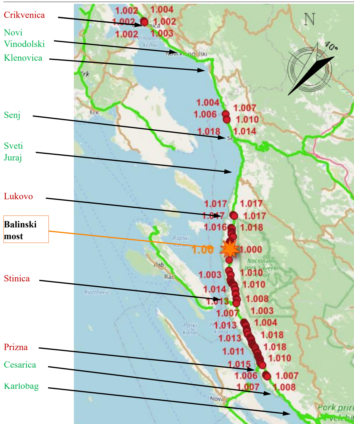
Slika 4.8 Točke sa većim brzinama vjetra od one na Balinskom mostu pri smjeru vjetra od 40°
