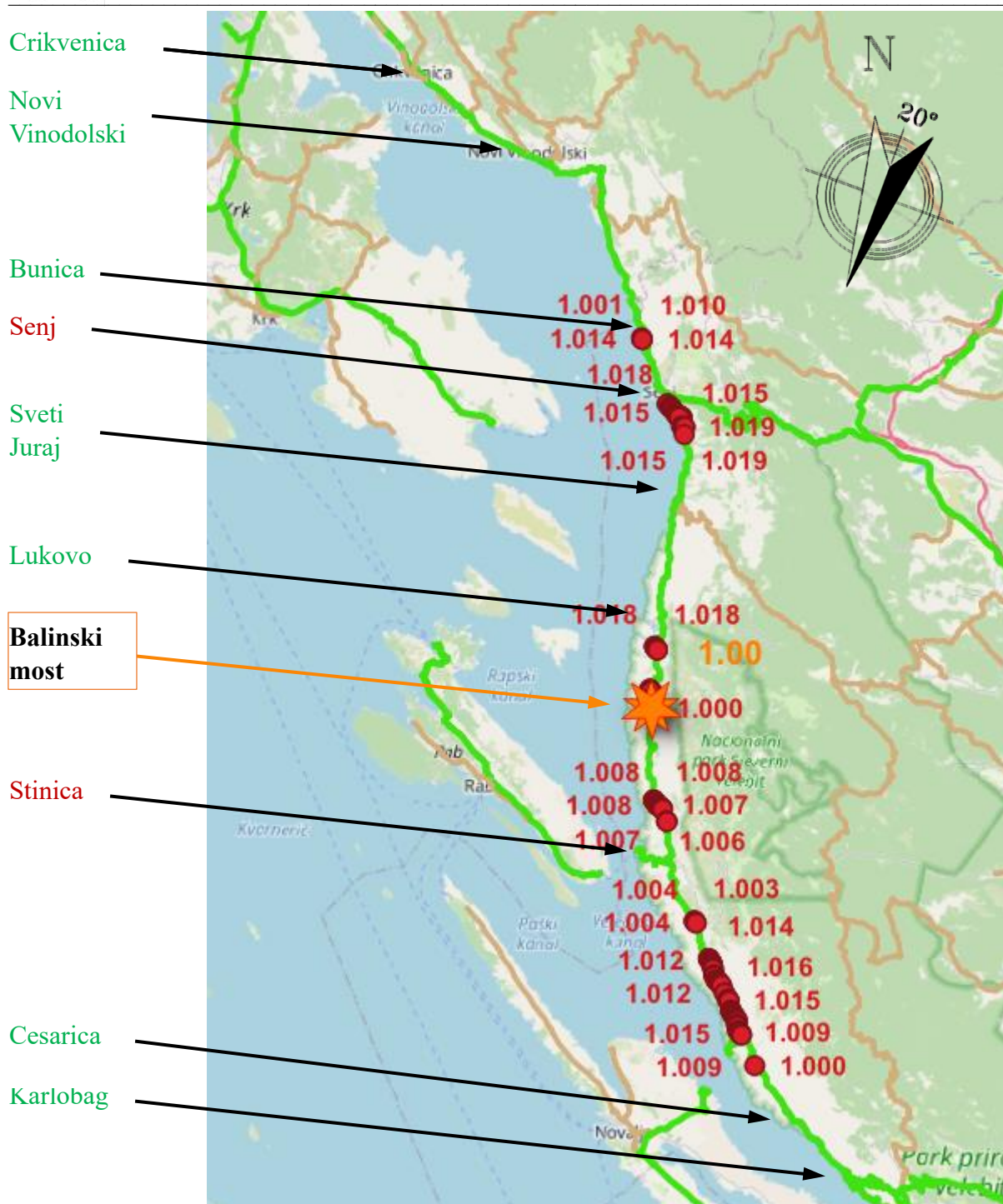
Slika 4.4 Točke sa većim brzinama od one na Balinskom mostu pri smjeru vjetra od 20°
