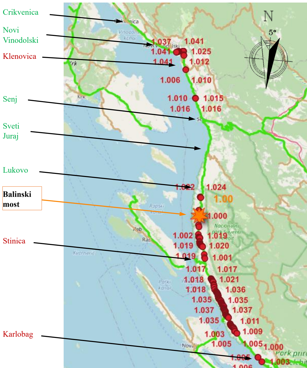
Slika 4.1 Točke sa većim brzinama od one na Balinskom mostu pri smjeru vjetra od 5°
