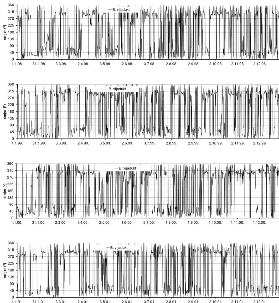
Slika 2.3 Slika 2.3 Vremenske serije smjera vjetra prema rezultatima numeričkog atmosferskog modela Aladin-Hr za razdoblje 1.1.1998.-1.1.2002. (4 km prostorna rezolucija i 3 satna vremenska rezolucija podataka), za poziciju točke 1 (Balinski vijadukt)
