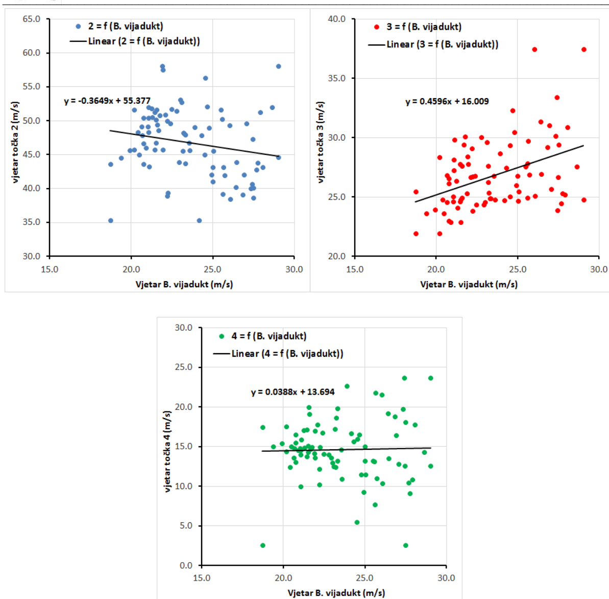
Slika 2.5 Odnosi smjera vjetra za točku 1 (Balinski vijadukt) i 2, 3, 4 (zaobalje) temeljem podataka iz modela Aladin-Hr za razdoblje 1.1.1998. – 1.1.2002. uz postavljeno ograničenje da trosatna brzina vjetra na poziciji Balinskog vijadukta bude veća od 19 m/s
