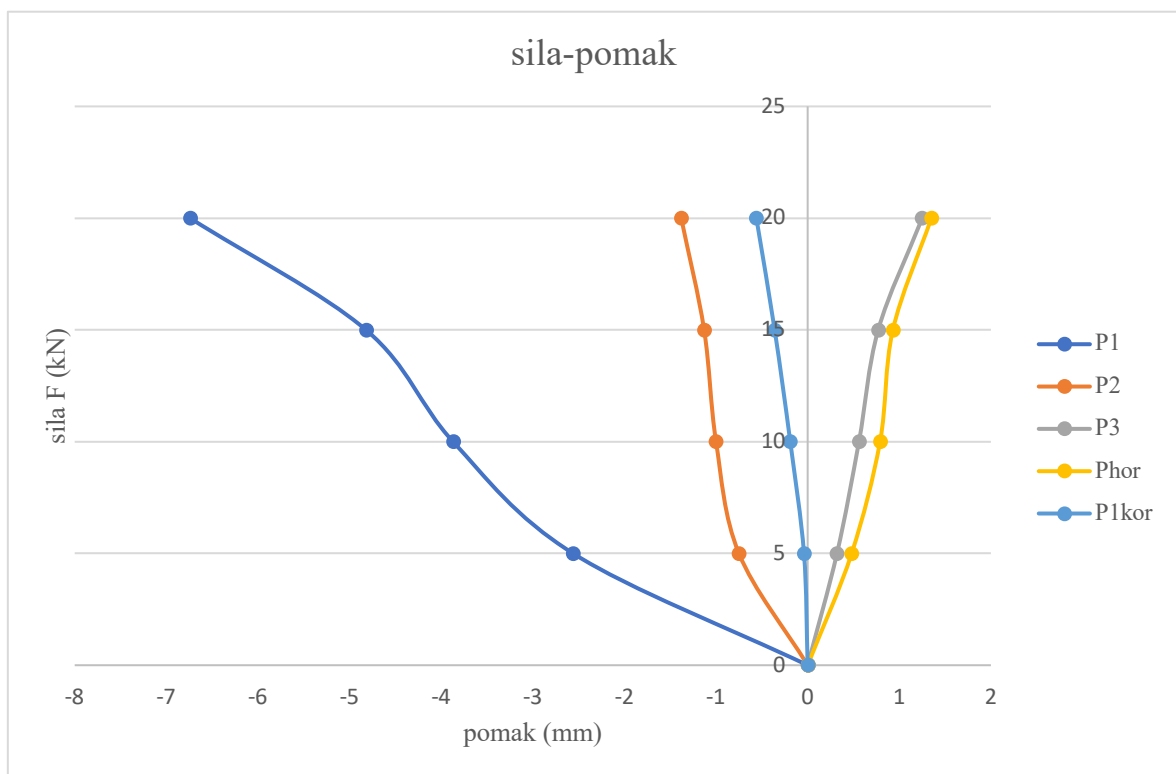
Slika 33 Dijagram sila-pomak
