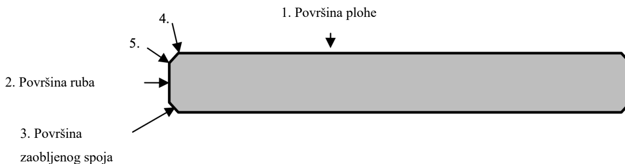
Slika 11 Predložena područja različitih grešaka na površini stakla (3)
