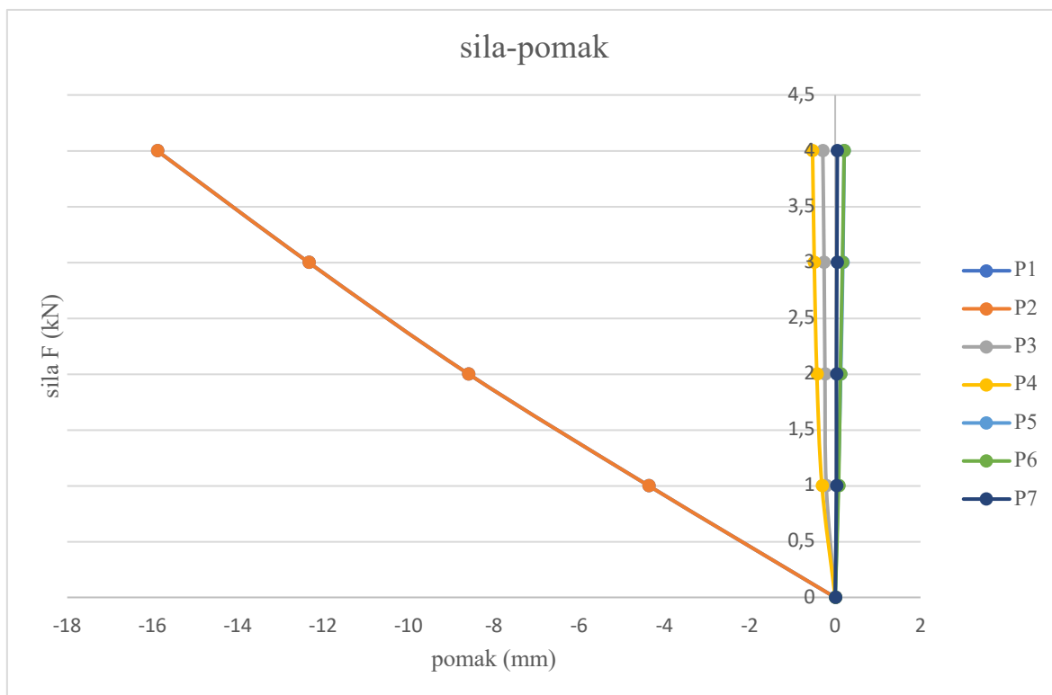
Slika 37 Dijagram sila-pomak
