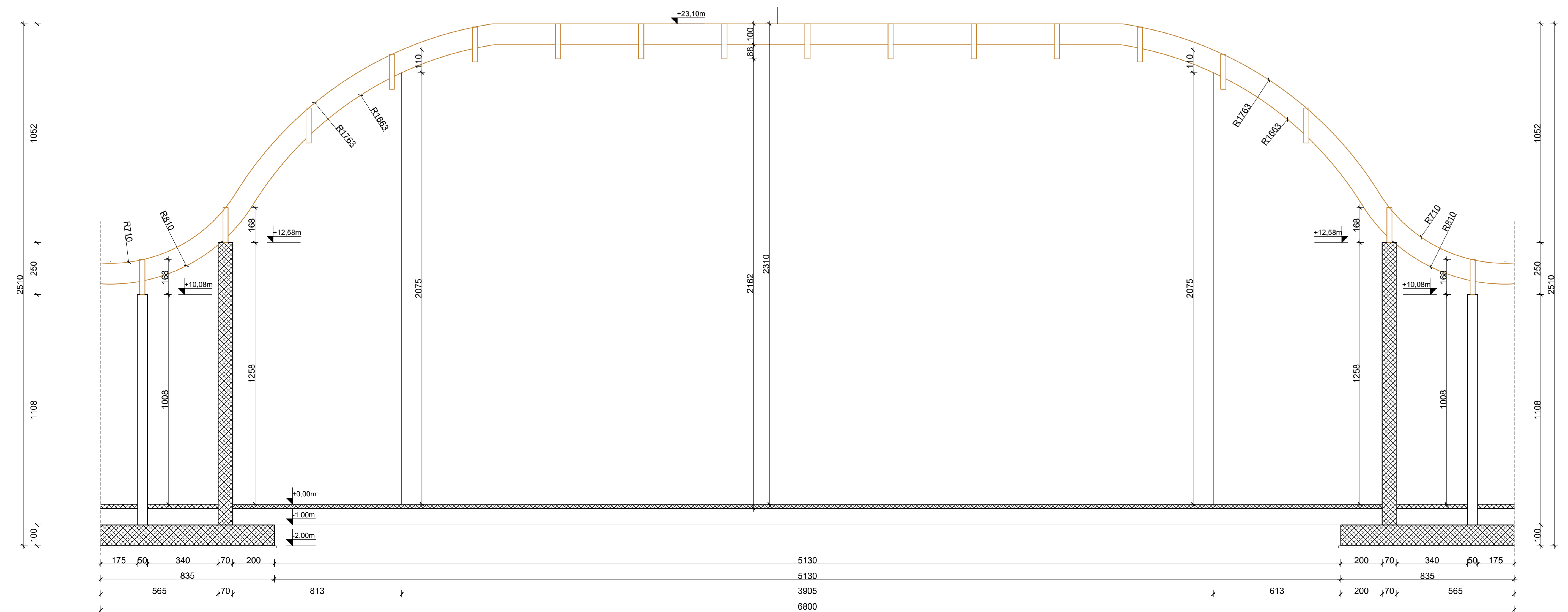
Presjek 1-1 M 1:100
