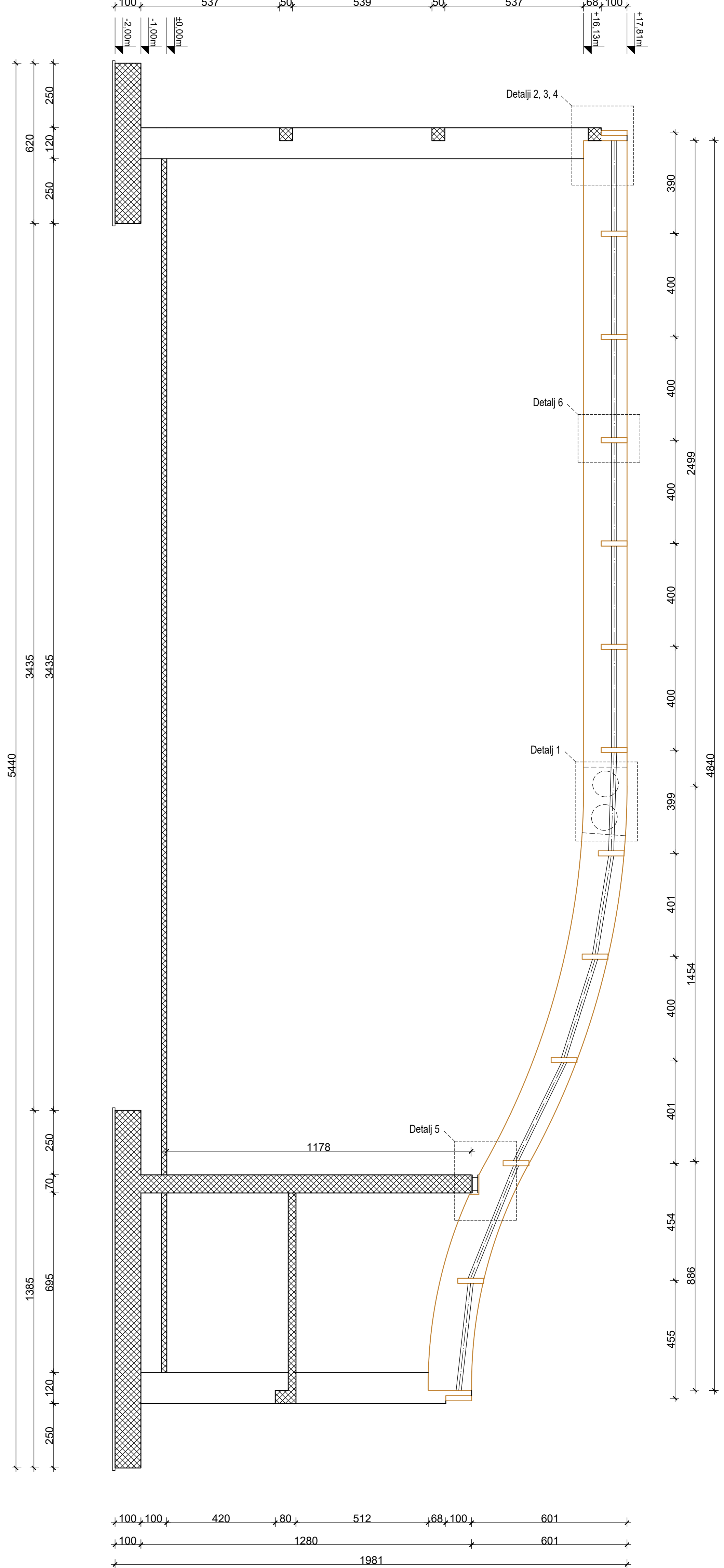
Presjek 2-2 M 1:100
