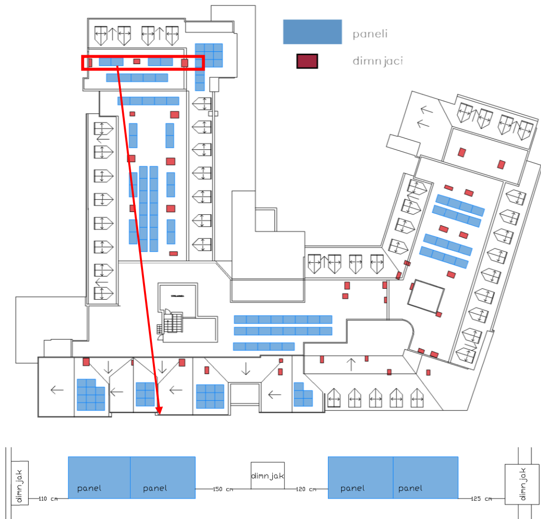
Slika 46 Položaj dimnjaka u odnosu na panele
