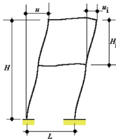
Slika 50. Shema ograničenja horizontalnih pomaka
