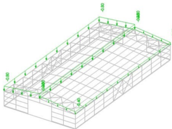
Slika 31.LC5 – snijeg lijeva stana krova
