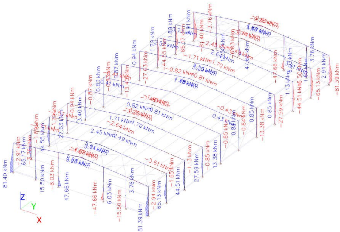
Slika 53. Rezne sile – Moment
