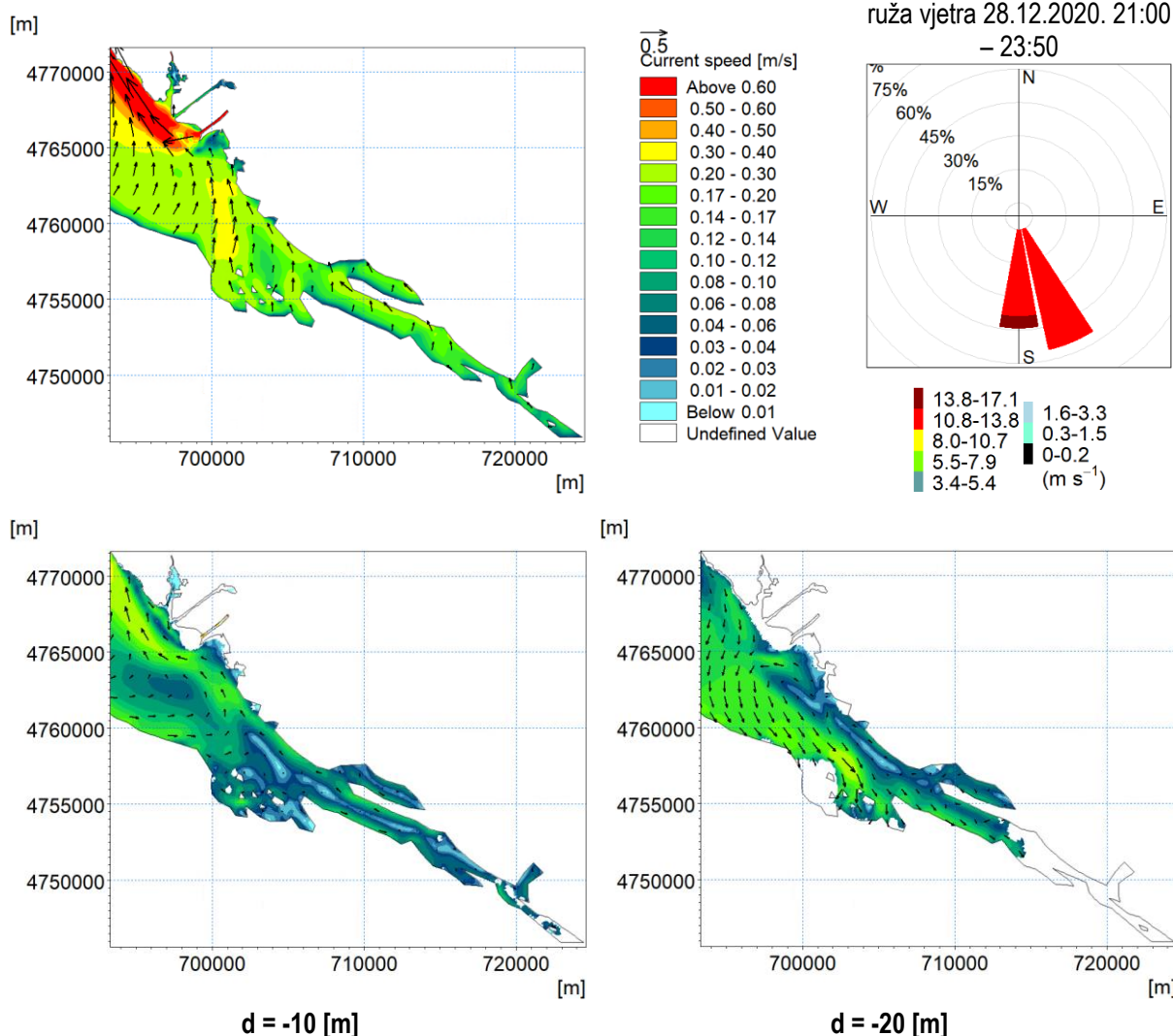
Slika 5-13 Polje brzine strujanja na dubinama -0,5 (gore lijevo), -10 (dolje lijevo) i -20 [m] (dolje desno) i ruža vjetera (gore desno) za vjetrovnu situaciju iz smjera S, v_{\max} = 14,8 [m·s -1 ], Q_{\text{Metković}} = 1016,0 [m 3 ·s -1 ], Q_{\text{Šipak}} = 44,4 [m 3 ·s -1 ] na datum 28.12.2020. u 23:00
