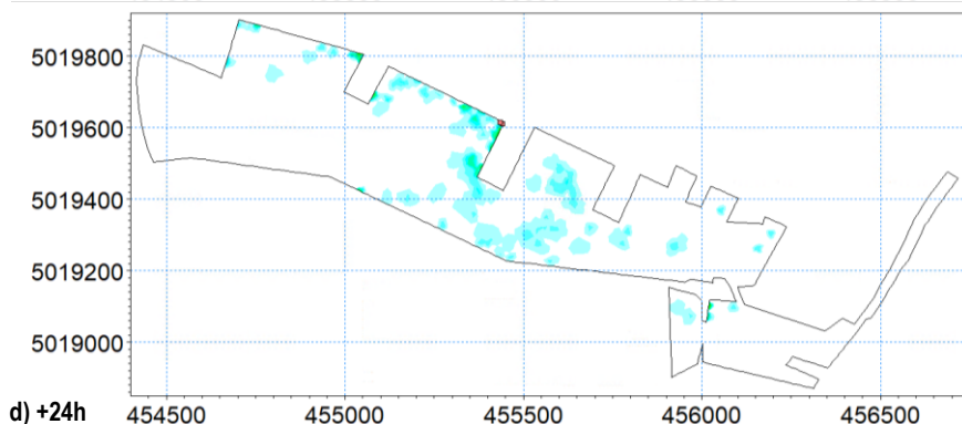
Slika 0-86 2D polja dinoflagelata raspršenih u stupcu mora izražena u [stanica·l -1 ] s prikazom modelskih čestica istaloženih na dnu 1, 6, 12 i 24 [h] (a, b, c, d) nakon unosa modelskih čestica u trenutku 15.10.2020. 12:00, ruža vjetrova na m.p. Rijeka (e) u razdoblju od 15.10.2020. u 12:00 do 16.10.2020. u 12:00
