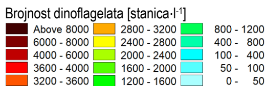
Slika 0-70 2D polja dinoflagelata raspoređenih u stupcu mora i istaloženih na dnu izražena u [stanica·l -1 ] 1, 6, 12 i 24 [h] (a, b, c, g) nakon unosa modelskih čestica u trenutku 30.10.2020. 09:00, ruža vjetrova na m.p. Ploče (d), protok na h.p. Šipak (e), protok i temperatura vode na h.p. Metković (f) u razdoblju od 30.10.2020. u 09:00 do 31.10.2020. u 09:00
