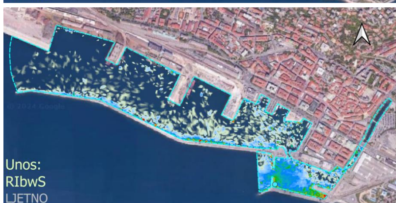
Slika 5-57 2D polja kopepoda raspršenih u stupcu mora i istaloženih na dnu za ZIMSKO i LJETNO simulacijsko razdoblje za unos modelskih čestica u prostornu domenu luke Rijeka na lokacijama „BazenSU-sredina“ i „RIbwS“ (podloga: Google satelit)
