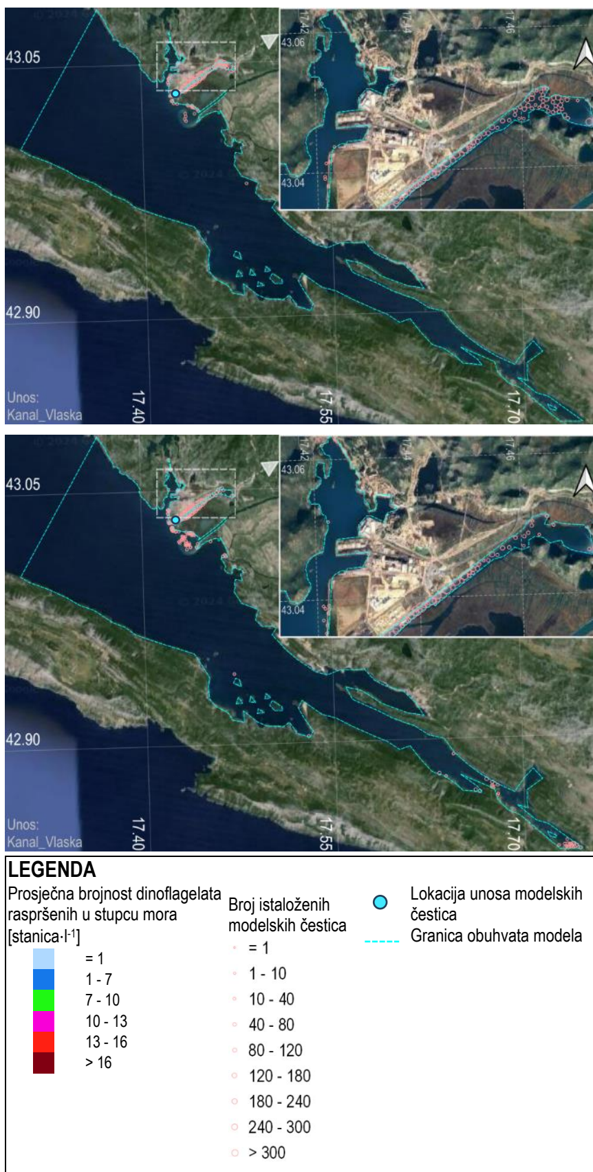
Slika 5-27 2D polja dinoflagelata raspršenih u stupcu mora i istaloženih na dnu za ZIMSKO (gore) i LJETNO (dolje) simulacijsko razdoblje za modelske čestice unesene u prostornu domenu šireg akvatorijalnog područja luke Ploče na lokaciji „Kanal_Vlaska“ (podloga: Google satelit)
