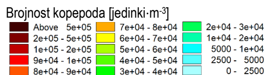
Slika 0-76 2D polja kopepoda raspršenih u stupcu mora i istaloženih na dnu izražena u [ \text{jedinki} \cdot \text{m}^{-3} ] 1, 6, 12 i 24 [h] (a, b, c, g) nakon unosa modelskih čestica u trenutku 30.10.2020. 09:00, ruža vjetрова na m.p. Ploče (d), protok na h.p. Šipak (e), protok i temperatura vode na h.p. Metković (f) u razdoblju od 30.10.2020. u 09:00 do 31.10.2020. u 09:00
