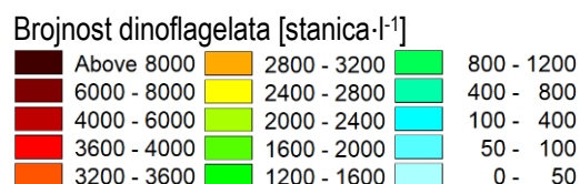
Slika 5-41 2D polja dinoflagelata raspšenih u stupcu mora i istaloženih na dnu izražena u [stanica- l^{-1} ] 1, 6, 12 i 24 [h] (a, b, c, g) nakon unosa modelskih čestica u trenutku 26.12.2020. 21:00, ruža vjetrova na m.p. Ploče (d), protok na h.p. Šipak (e), protok i temperatura vode na h.p. Metković (f) u razdoblju od 26.12.2020. u 21:00 do 27.12.2020. u 21:00
