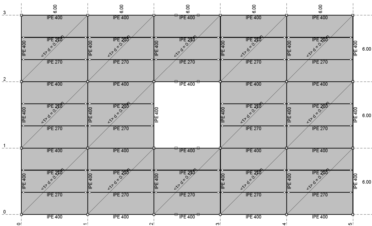
Nivo: POZ 400 - Strop 3. kata [14.00 m]
