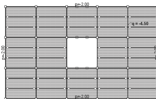
Nivo: POZ 500 - Strop 4. kata [17.50 m] Opt. 2: G2 - Dodatno stalno opterećenje
