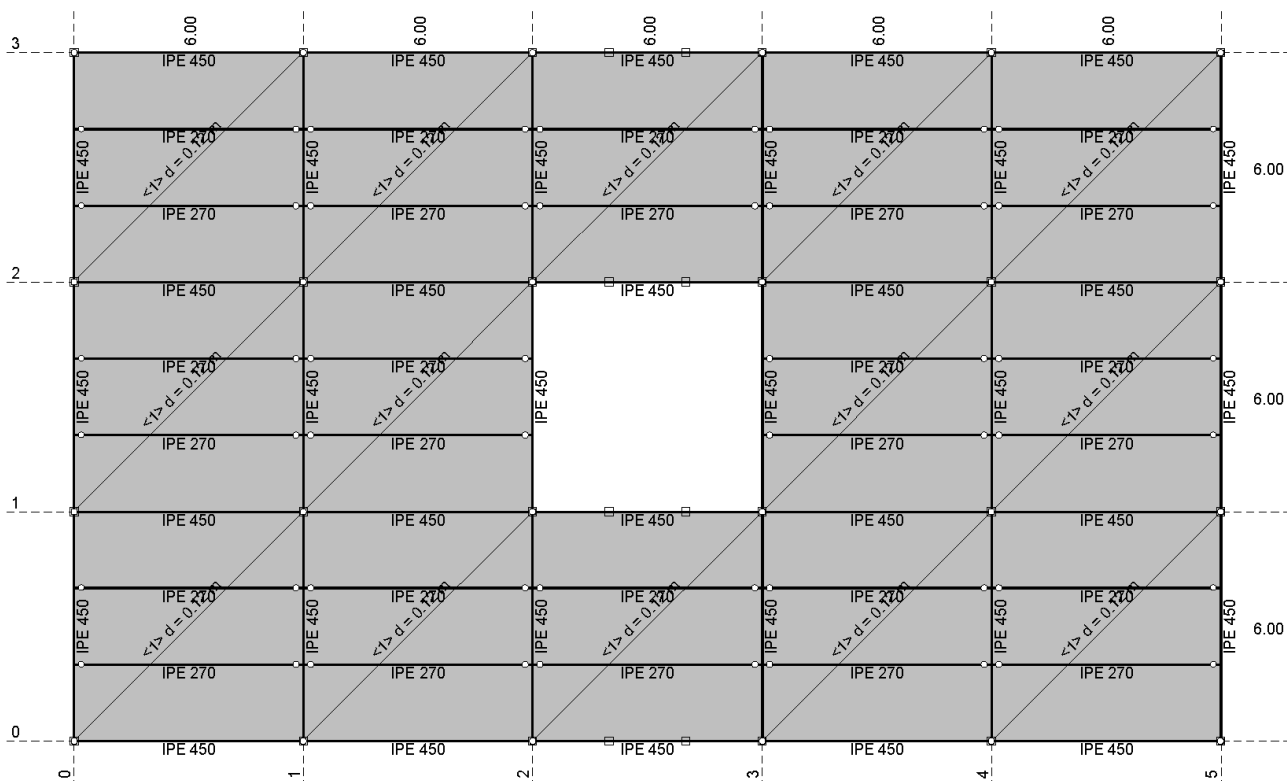
Nivo: POZ 200 - Strop 1. kata [7.00 m]
