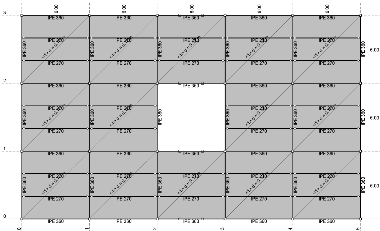
Nivo: POZ 500 - Strop 4. kata [17.50 m]
