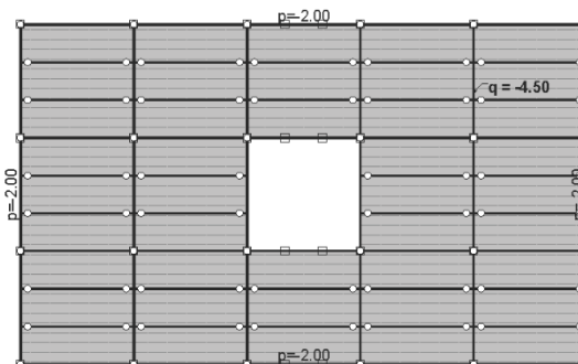
Nivo: POZ 300 - Strop 2. kata [10.50 m] Opt. 2: G2 - Dodatno stalno opterećenje
