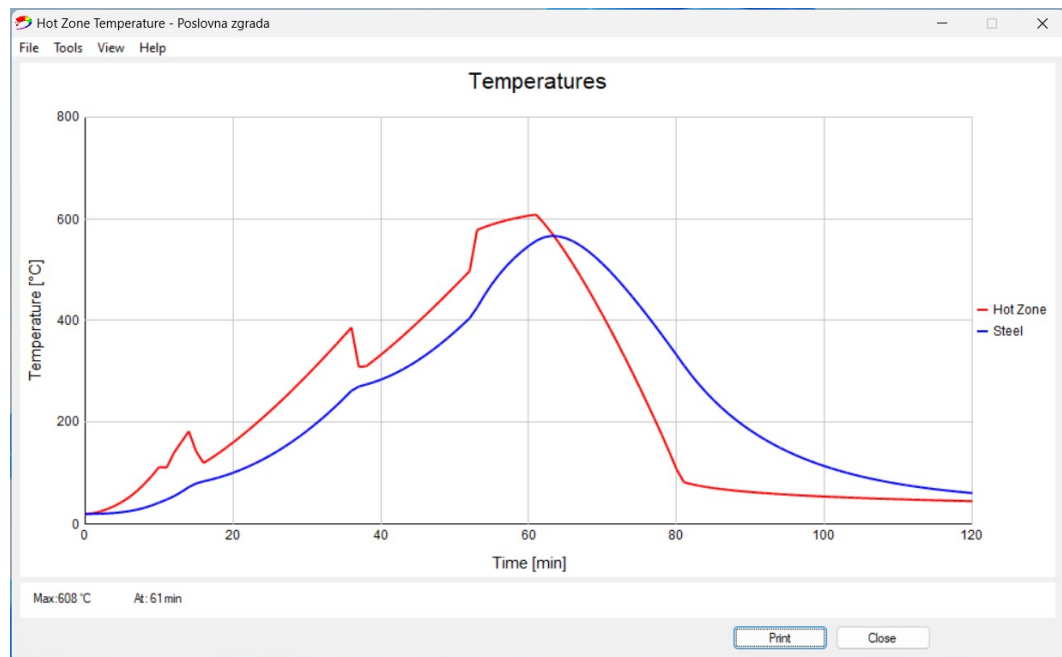
Slika 59 Scenarij 4 – Sa aktivnom zaštitom od požara u vidu detektora dima
