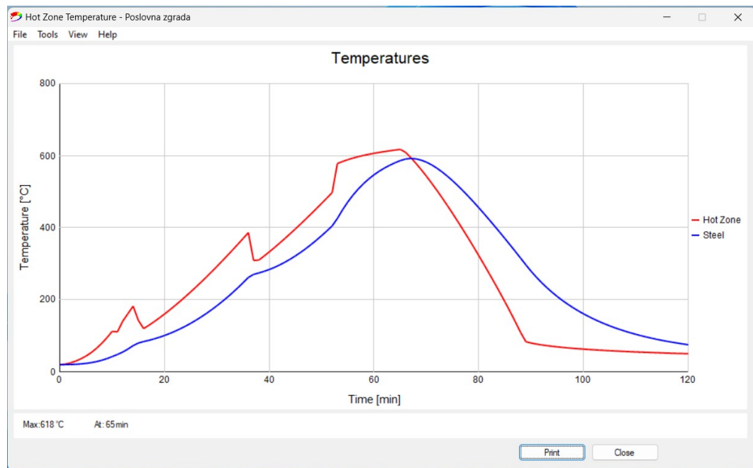
Slika 58 Scenarij 3 – Sa aktivnom zaštitom od požara u vidu detektora topline
