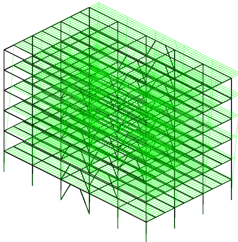
Izometrija Forma osciliranja: 1/10 [T=1.1495sec / f=0.87Hz]
