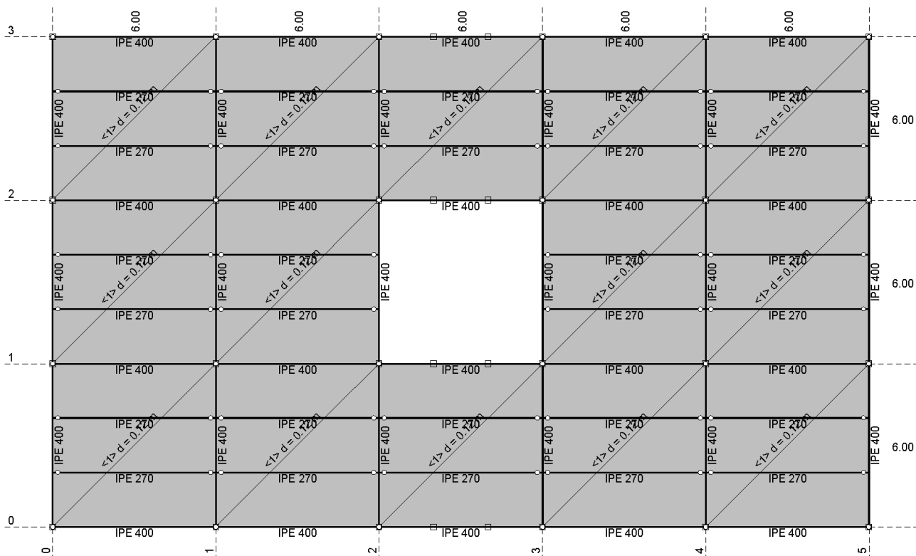
Nivo: POZ 300 - Strop 2. kata [10.50 m]
