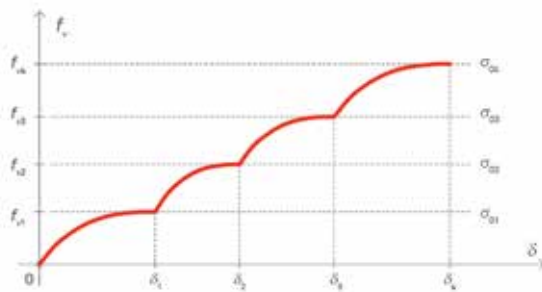
Slika 22. Dijagram zavisnosti pomaka \delta i posmične čvrstoće zida f_v [6]
