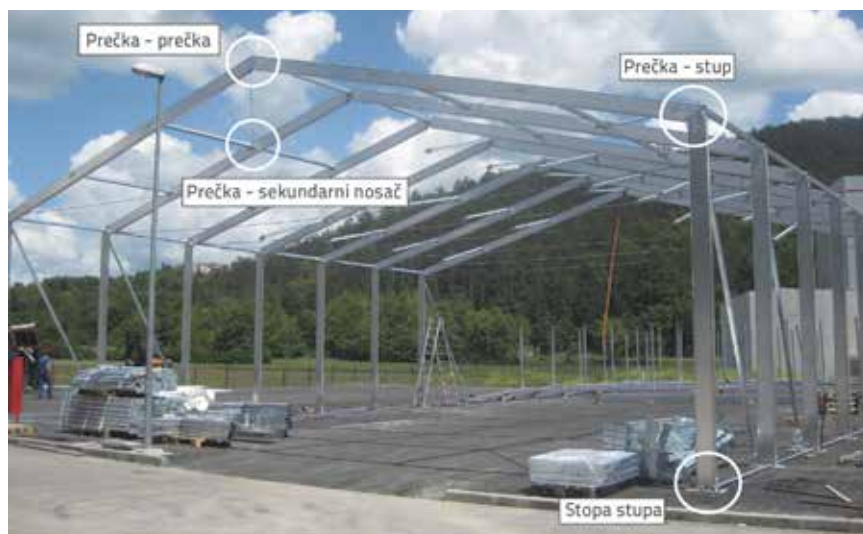
Slika 8. Karakteristični priključci montažne aluminijske hale
