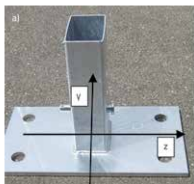
Slika 9. Varijante stope stupa
