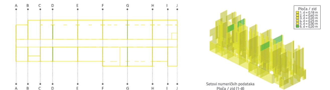
Slika 2. Tlocrt trećeg kata i 3D model konstrukcije s oznakama zidova koji se izvode betonom s recikliranim agregatom
