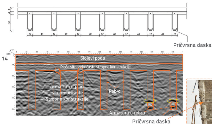
Slika 12. Rekonstrukcija sitnorebraste stropne konstrukcije georadarom na osnovi radargrama 14
