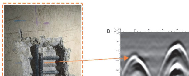
Slika 6. Određivanje rasporeda armature stupa s jedne strane
