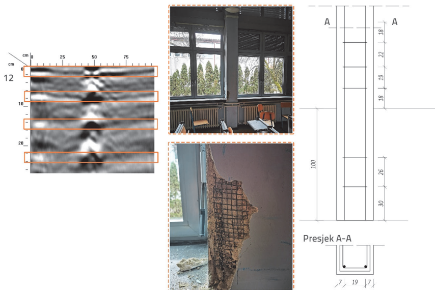
Slika 10. Radargram 12 (lijevo), Rabicova mreža stupa (sredina) i nacrt rasporeda armature (desno)
