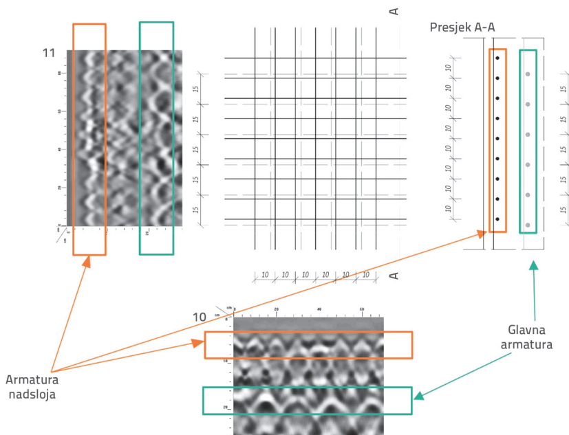
Slika 9. Određivanje položaja armature nadsloja i glavne armature stropne ploče
