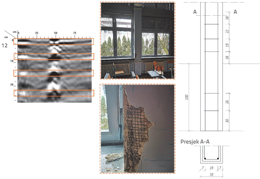
Slika 10. Radargram 12 (lijevo), Rabičova mreža stupa (sredina) i nacrt rasporeda armature (desno)
