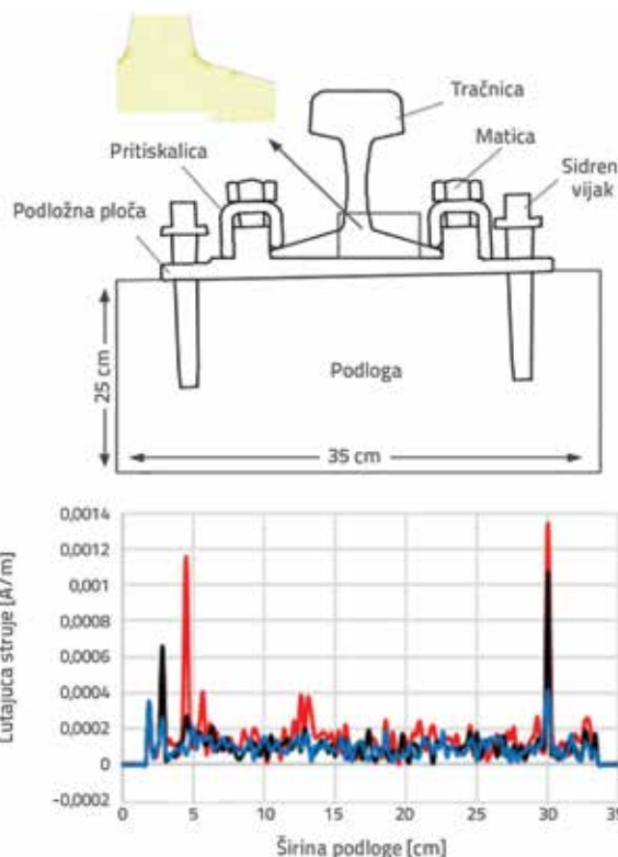
Slika 27. Raspodjela lutajućih struja na mjestu pričvršćenja tračnice kod različitih vrijednosti električnog otpora podloge [49]
