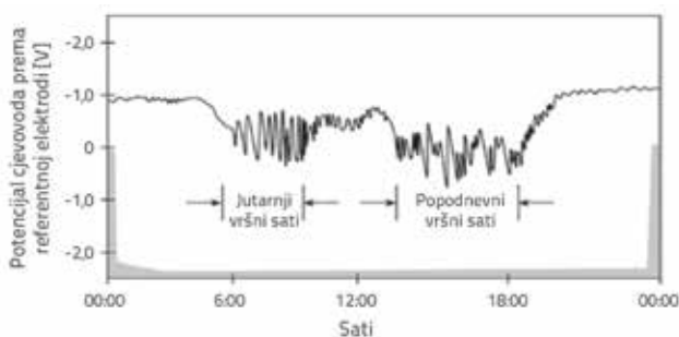
Slika 8. Potencijal cjevovoda mjereno u periodu od jednog dana [29]
