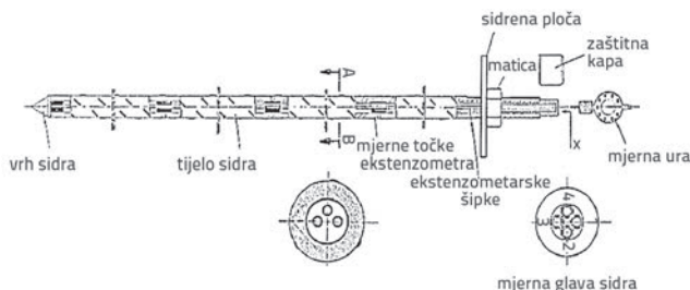
Slika 4. Elementi mjernog sidra, modificirano iz [12]
