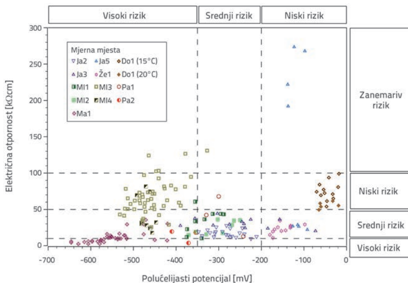
Slika 10. Korelacija između polučelijastog potencijala i električne otpornosti za sva mjerna mjesta
