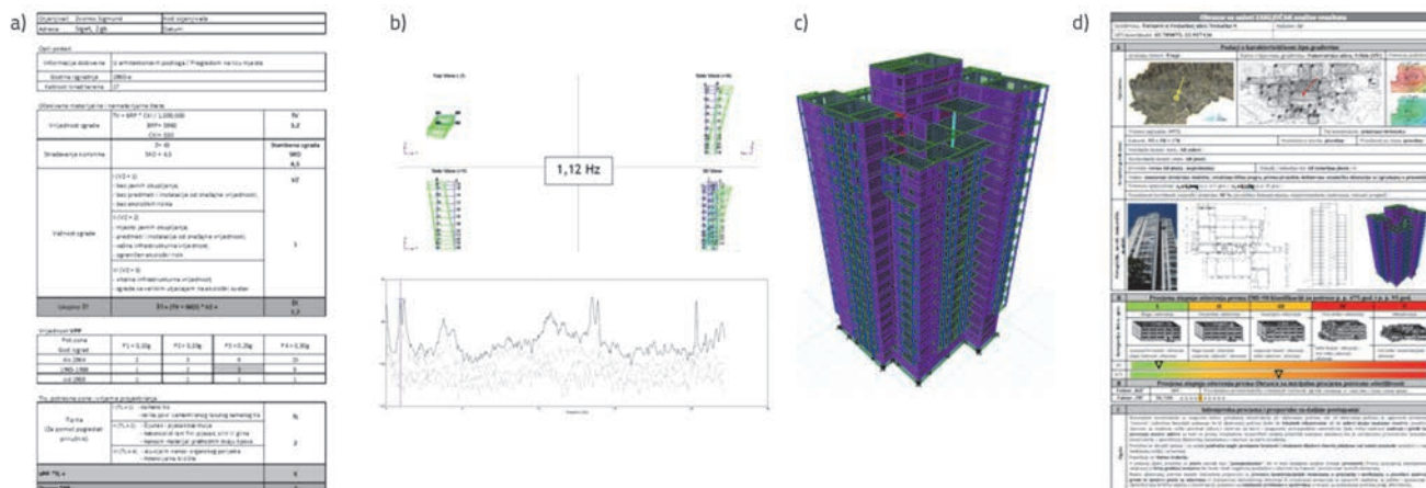
Slika 16. Pristup detaljnoj analizi postojeće građevine na temelju prikupljenih podataka: a) obrazac za inicijalnu procjenu potresne oštećljivosti; b) eksperimentalna istraživanja dinamičkih parametara; c) numerički model; d) obrazac sa sažetim prikazom rezultata analize [83]
