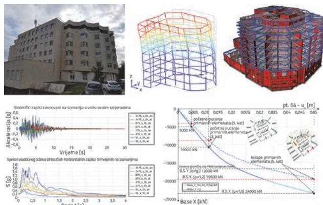
Slika 24. Detaljna analiza Opće bolnice u Dubrovniku: a) fotografija analizirane građevine, b) rezultati eksperimentalnih mjerenja ambijentalnih vibracija, c) numerički model, d) zapisi ubrzanja u vremenu, e) krivulja kapaciteta nosivosti zgrade [101]
