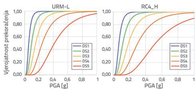
Slika 21. Primjeri krivulja vjerojatnosti oštećenja za tipove nosivih sustava URM_L i RC4_H
