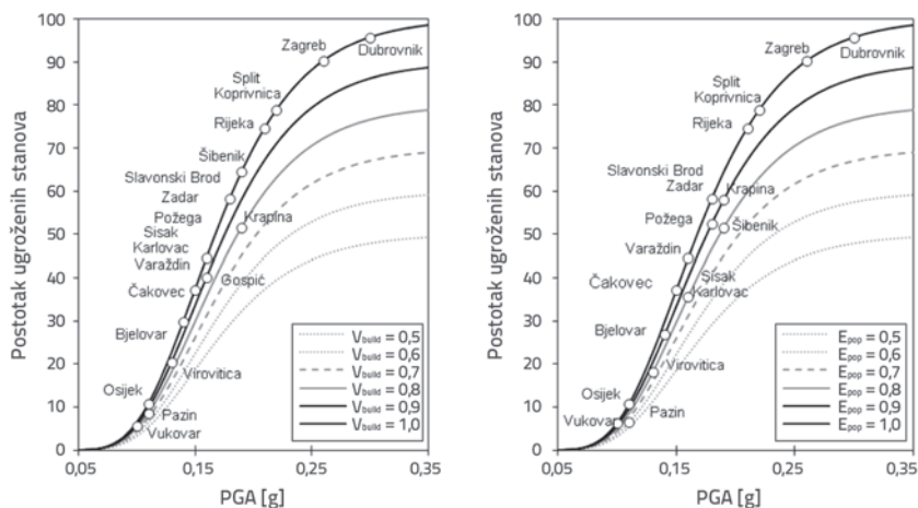
Slika 17. Modeli predviđanja potresnog rizika za Hrvatsku [87]
