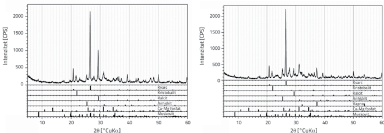
Slika 4. XRD difraktogram i mineraloški sastav pepela dobivenog spaljivanjem mulja s UPOV-a Karlovac pri 800 °C (lijevo) i 900 °C (desno)
