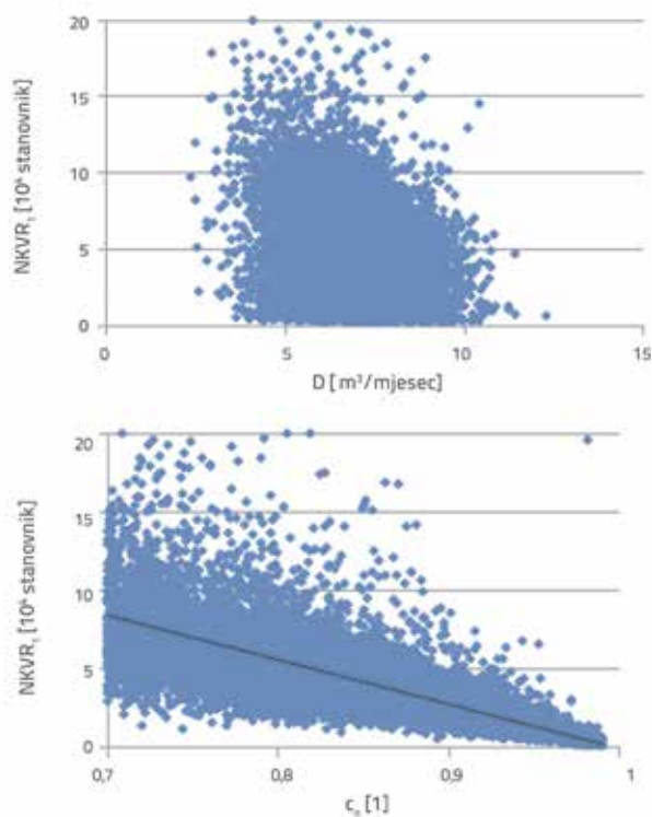
Slika 7. Dijagrami raspršenosti parametara D i c_n u odnosu na NKVR_1
