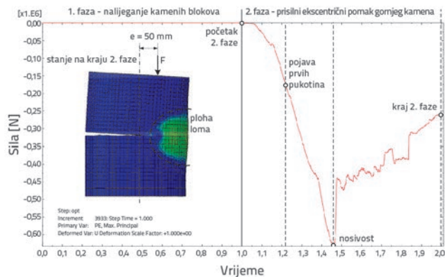
Slika 19. Dijagram sile i pseudo-vremena na uzorku bez olovnoga umetka
