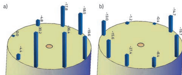
Slika 12. Faza ispitivanja pri centričnoj sili od 500kN i ekscentričnoj sili od 200kN za uzorak K5 s olovnim umetkom: a) vrijednosti naprezanja u VS [MPa], b) vrijednosti naprezanja u DS [MPa]
