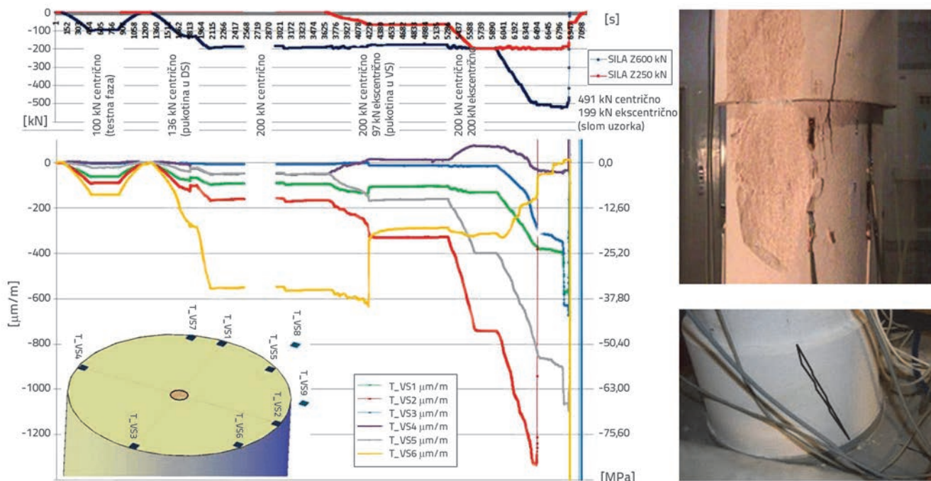
Slika 6. Dijagram ispitivanja uzorka K3 – relativne deformacije (naprezanja) u vremenu s prikazom tijeka unosa opterećenja za mjerno mjesto vrh stupa (VS) s fotografijama otvaranja pukotina u VS i DS
