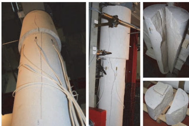
Slika 15. Pukotina s obje strane uzorka K5 bez olovnoga umetka te rascijepljenje tijela i baze stupa nakon rastavljanja
