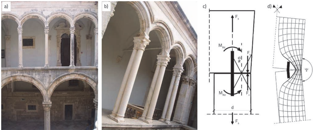
Slika 2. a) Tradicijski kameni stupovi; b) Udvojeni stupovi na katu Kneževa dvora u Dubrovniku; c) Model ponašanja spoja s unutarnjim silama i napreznjima [7]; d) Razdioba trajektorija napreznja [6]
