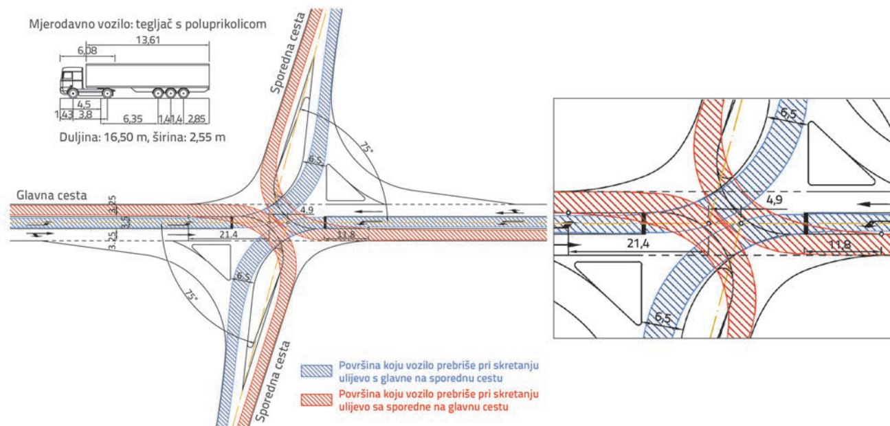
Slika 2. Provjera provoznosti četverokrakog raskrižja s razmaknutim osima sporedne ceste, oblikovanom prema normi [15] i smjericama [16], za kut križanja od 75°
