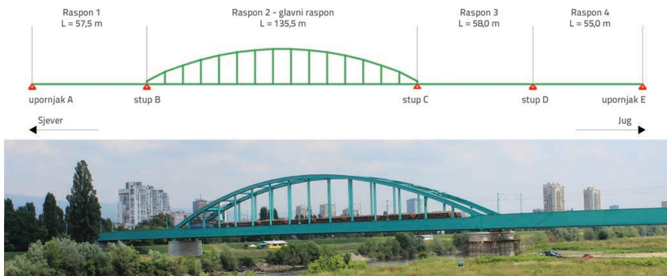
Slika 1. Željeznički most "Sava" – uzdužna dispozicija (gore) i fotografija mosta (dolje)
