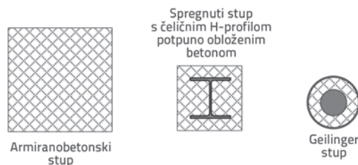
Slika 3. Usporedba različitih poprečnih presjeka stupova za isto opterećenje
