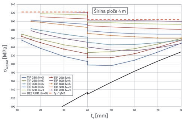
Slika 6. Računsko naprezanje otpornosti na izbočivanje za ukrućene ploče širine 4 m
