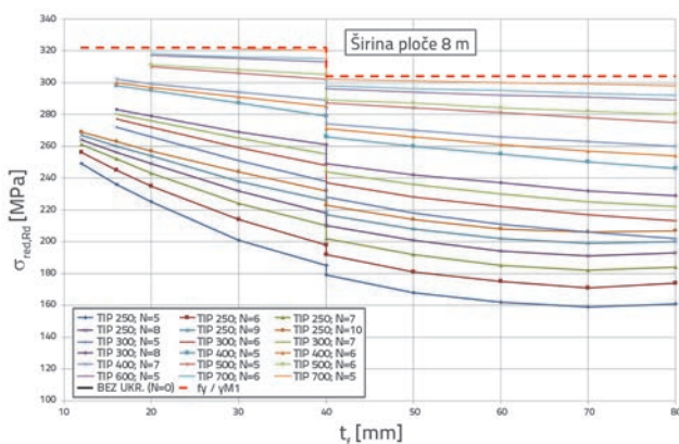
Slika 8. Računsko naprezanje otpornosti na izbočivanje za ukrućene ploče širine 8 m
