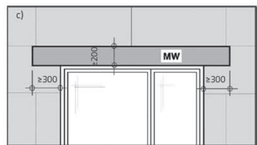
Slika 5. Protupožarna barijera: a) postavljena na uzorku EM_2; b) shema - presjek [14]; c) shema - pogled [14]
