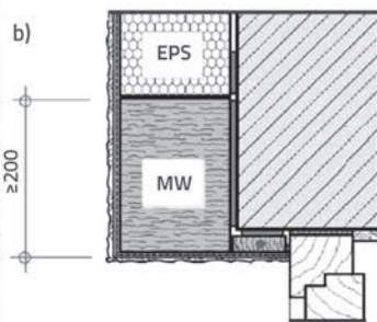
Slika 5. Protupožarna barijera: a) postavljena na uzorku EM_2; b) shema - presjek [14]; c) shema - pogled [14]
