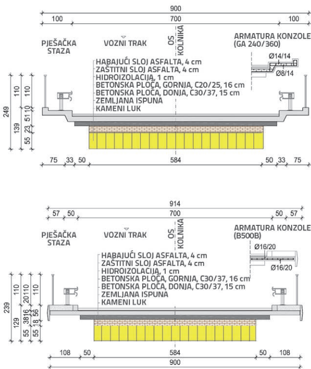
Slika 7. Poprečni presjek postojećeg mosta (gore) i predlog sanacije kolničke ploče (dolje)
