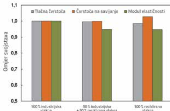
Slika 13. Utjecaj udjela recikliranih čeličnih vlakana na svojstvo tlačne i vlačne čvrstoće te modula elastičnosti
