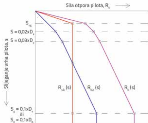
Slika 8. Karakteristična krivulja nosivost – slijeganje vrha pilota (DIN 1054) [33]
