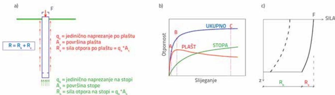
Slika 1. Prikaz prijenosa sila u tlačno opterećenom pilotu
