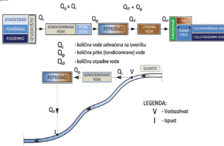
Slika 4. Sustav s jednokratnom uporabom vode i bez pročišćavanja otpadnih voda
