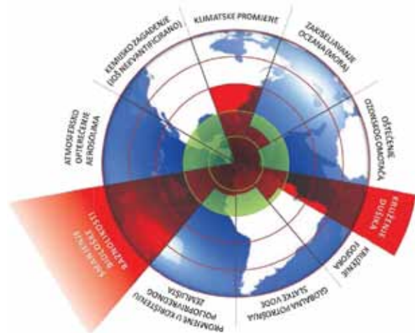
Slika 2. Planetarne granice
